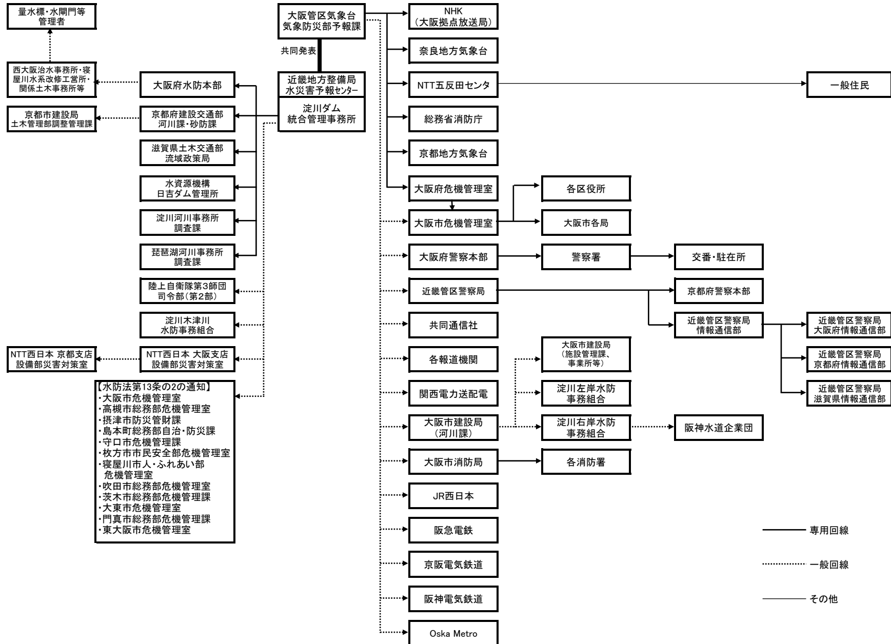
淀川洪水予報伝達系統図
