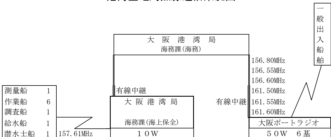
港湾基地局無線通信系統図
