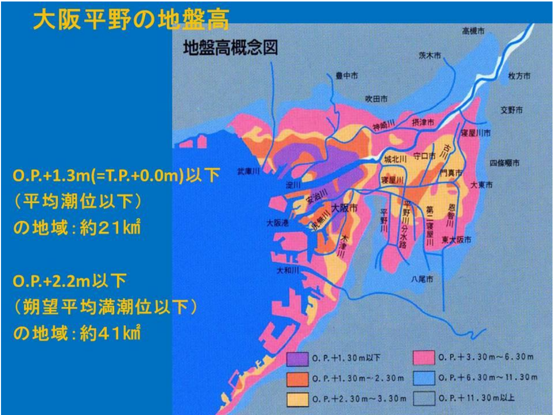
図 大阪平野の地盤高 出典：大阪府 「[津波・高潮ステーション]海より低いまち大阪」 ( http://www.pref.osaka.lg.jp/nishiosaka/tsunami/tsuna-symbol.html ) より
