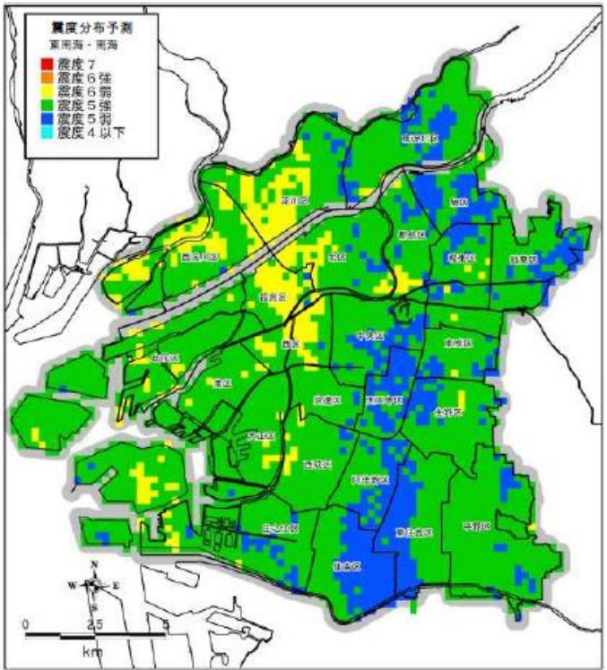
図 予測震度（東南海・南海地震）
