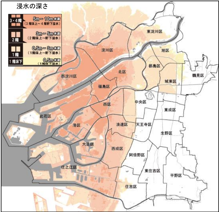
図 大阪市域に高潮が発生した場合の浸水想定区域図 出典：令和2年8月 大阪府港湾局公表浸水想定区域図を一部加工
