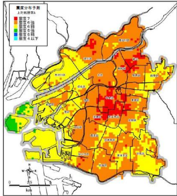
図 予測震度（上町断層帯地震）
