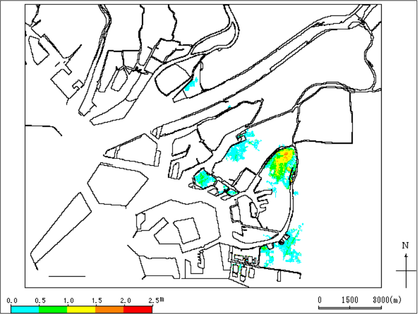
図 東南海・南海地震津波浸水予測
