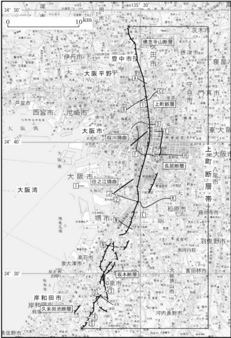
図 市域の活断層
