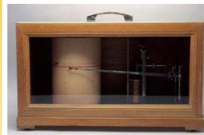
アネロイド型自記気圧計
