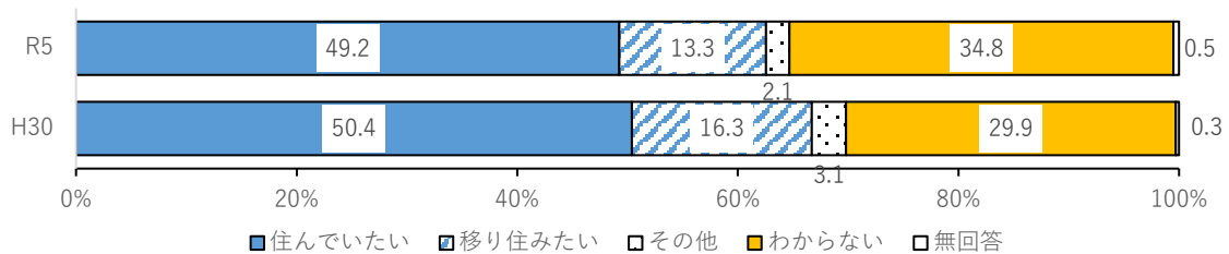
図49 将来ずっと大阪市に住んでいたい (15～39歳) (大阪市)
