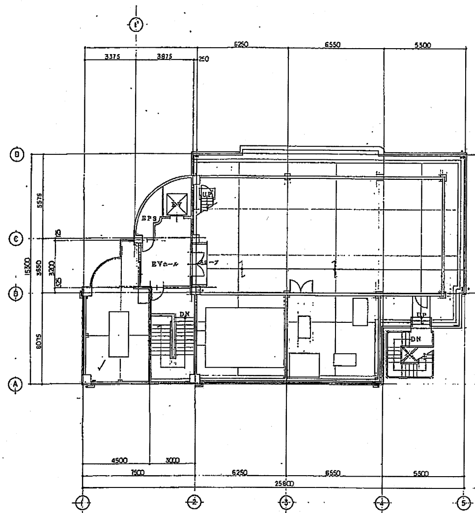
6階平面図 S: 1/250
