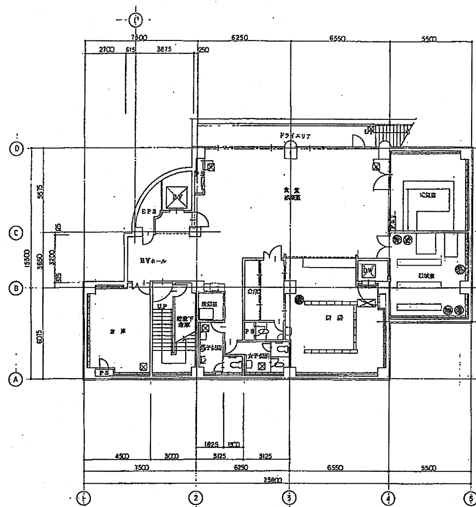
地階平面図 S: 1/250
