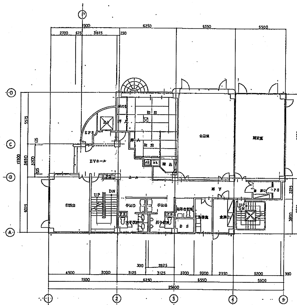
4階平面図 S: 1/250
