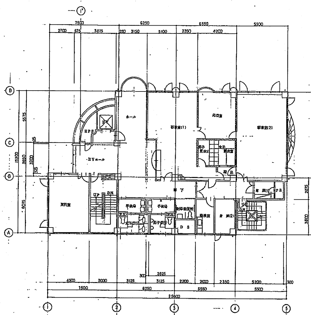
3階平面図 S: 1/250
