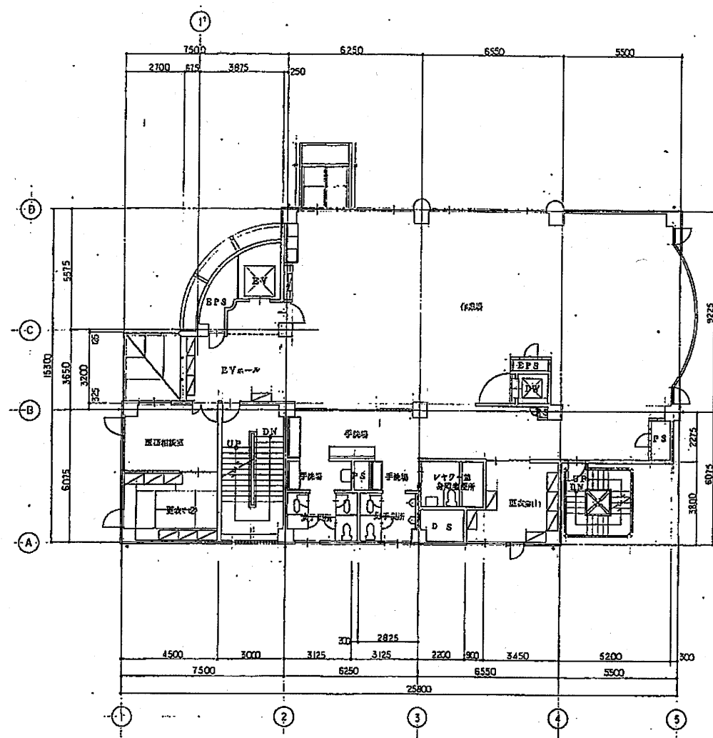
2階平面図 S: 1/250
