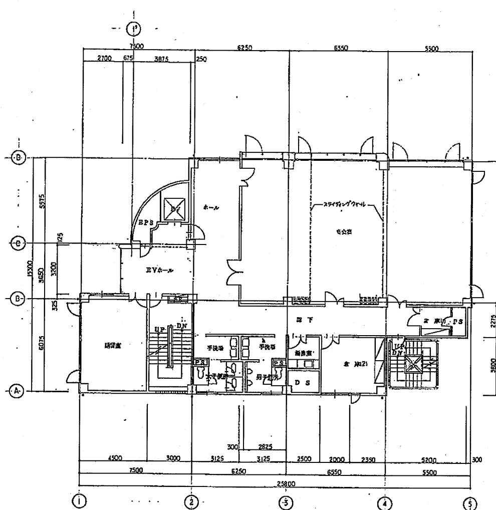
5階平面図 S: 1/250
