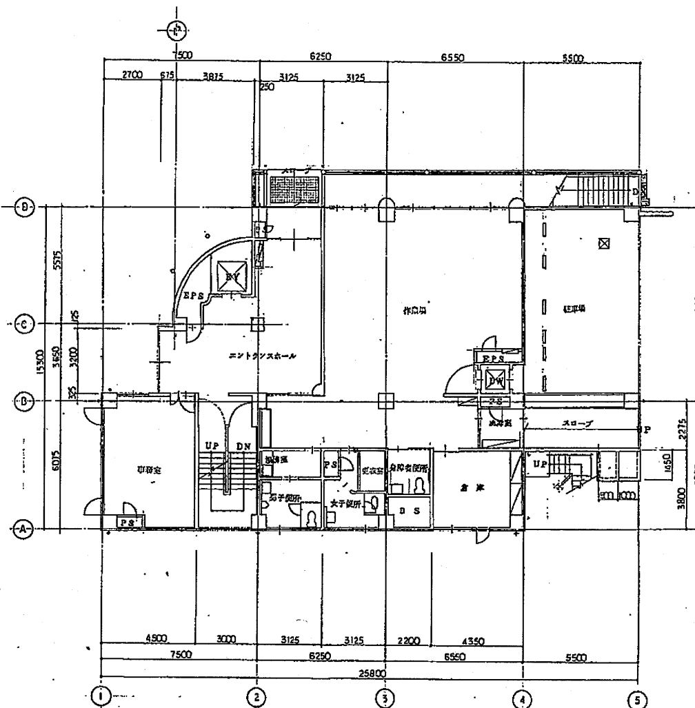
1階平面図 S: 1/250
