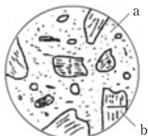
火成岩A
