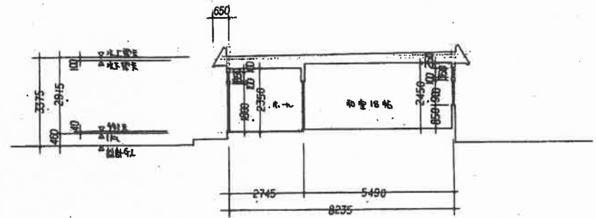
断面图 1/100
