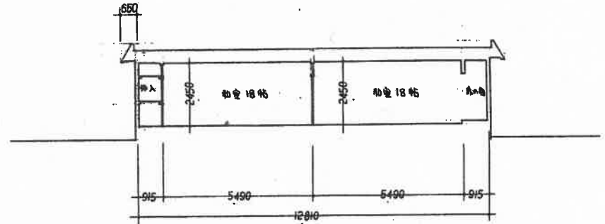
断面图 1/100
