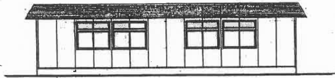
东面立面图 1/100
