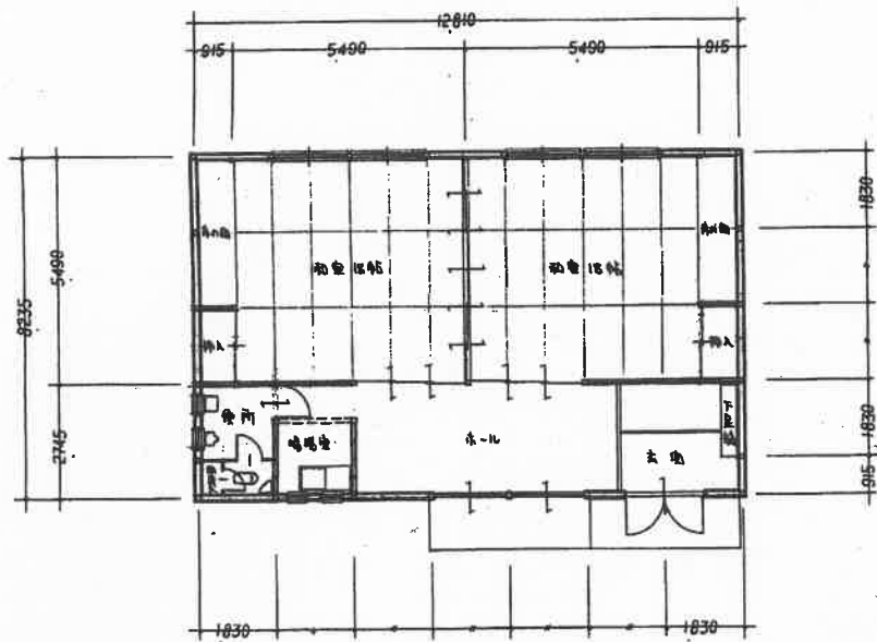
平面图 1/100
