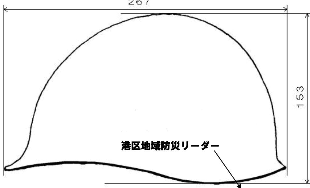
側面図
