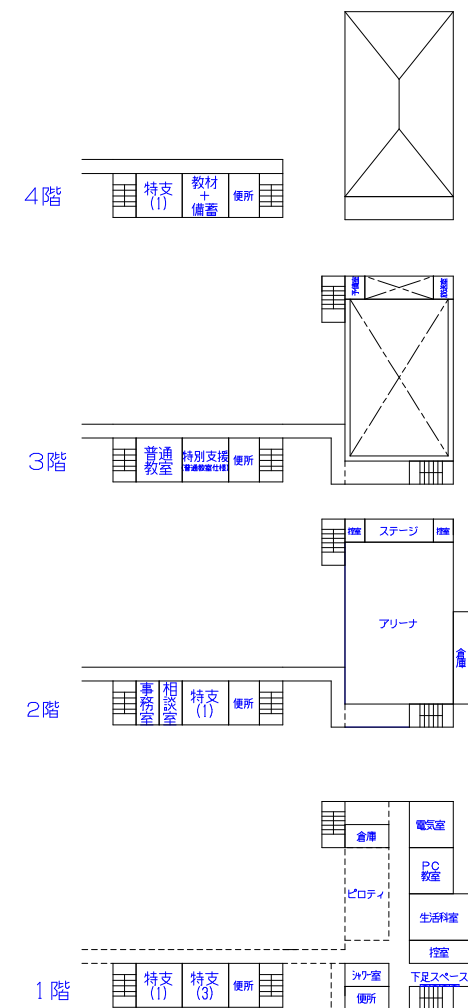
【平面図】
