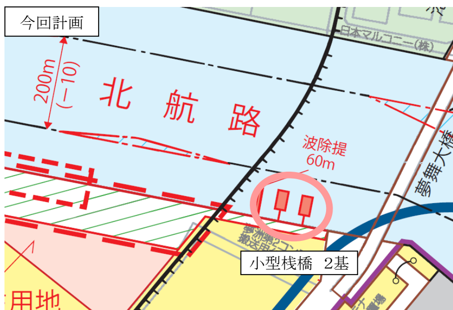
図 2－1 夢洲地区旅客船埠頭計画
