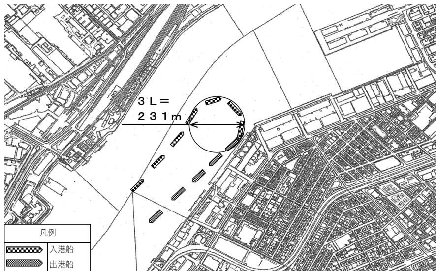
図 2 - 1 - 4 操船例図
