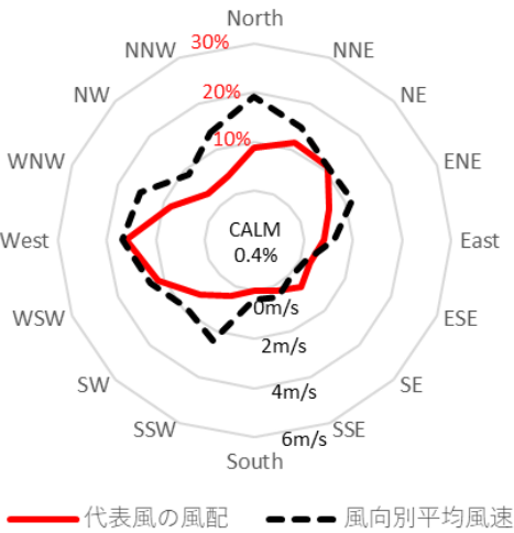
風の頻度分布図 (大阪港)
