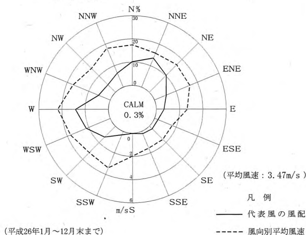
風の頻度分布図 (大阪港)
