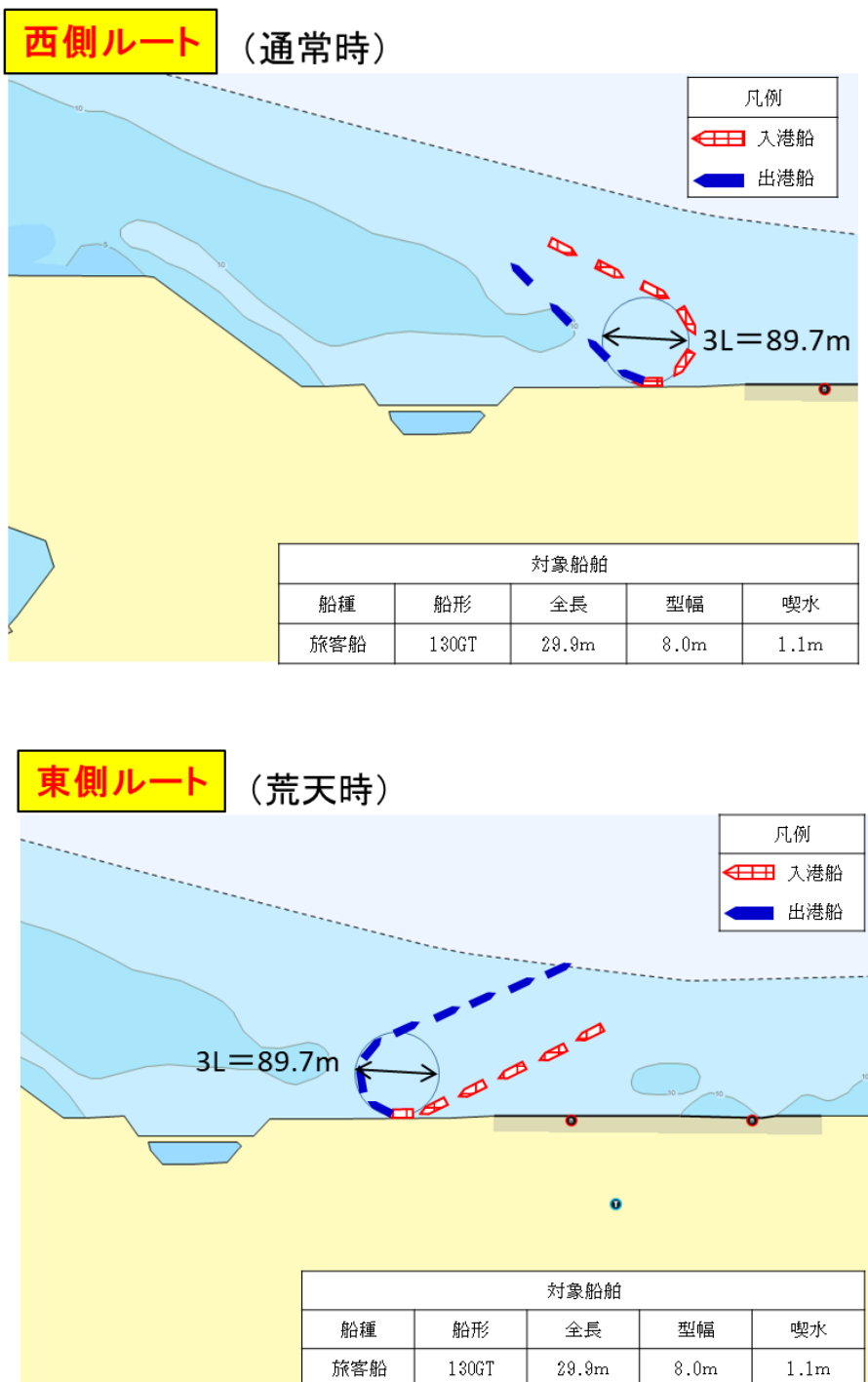
図 2 - 1 - 2 操船例図
