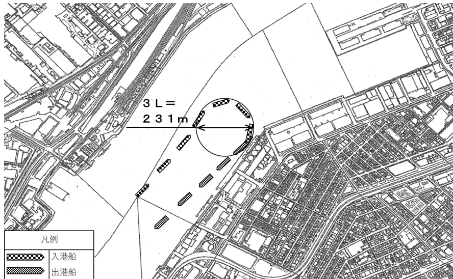
図 2 - 1 - 4 操船例図
