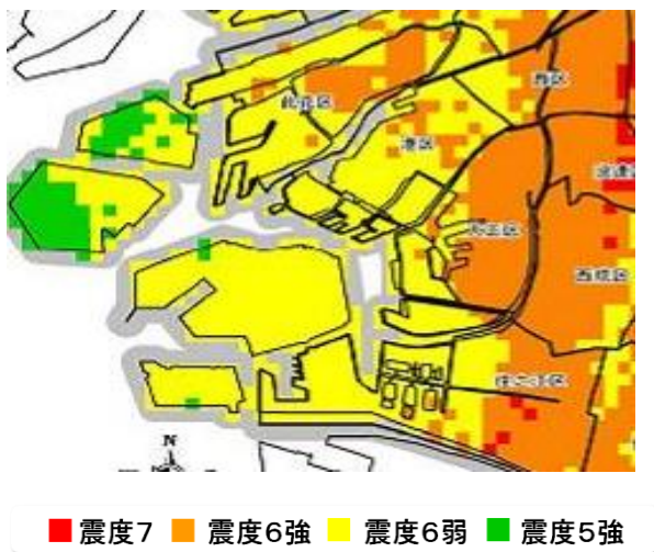
図 3-1 震度分布図
