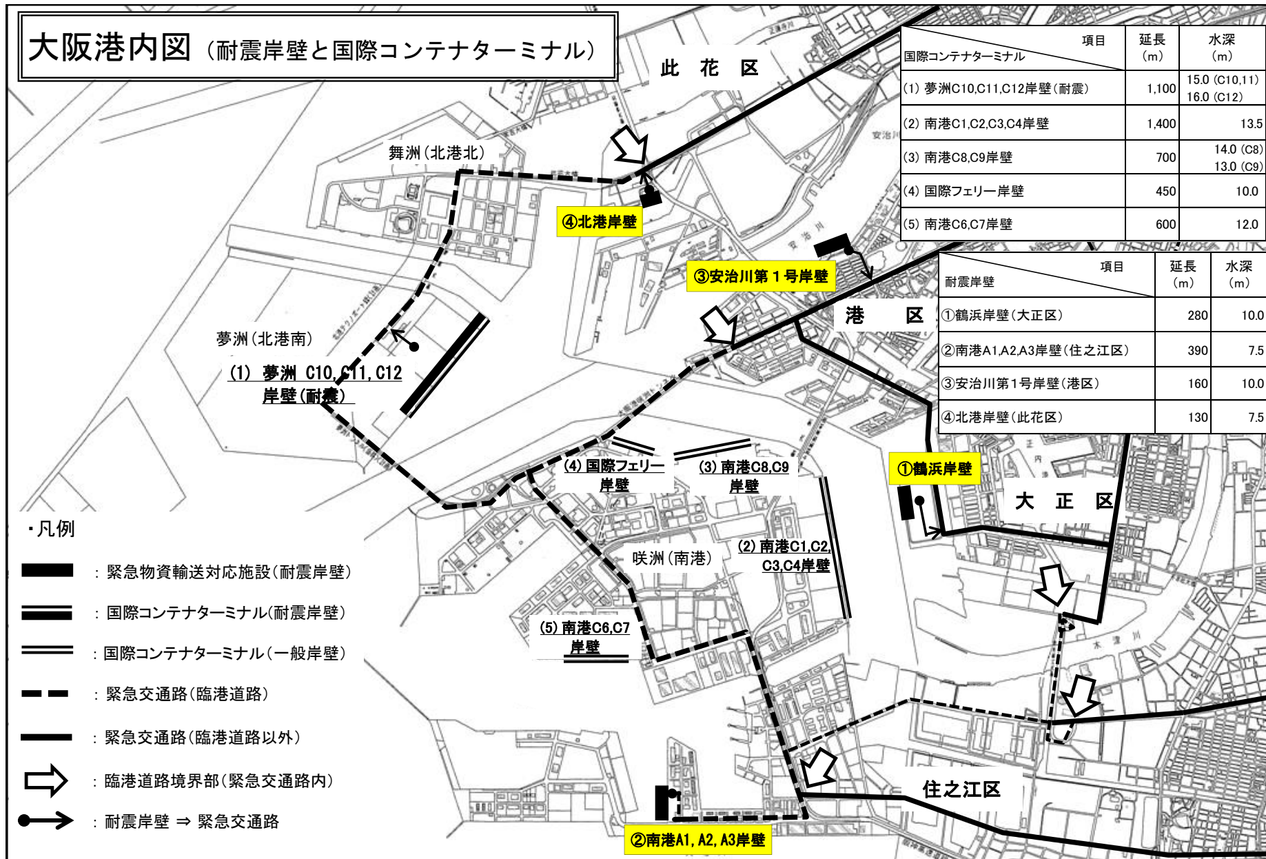
図 3-3 大阪港の耐震岸壁等位置図
