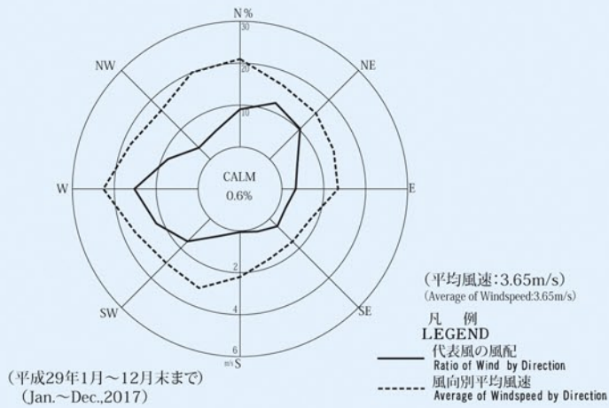
風の頻度分布図 (大阪港) Wind Frequency Distribution Diagram WIND ROSE
