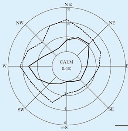
風の頻度分布図 (大阪港) Wind Frequency Distribution Diagram WIND ROSE
