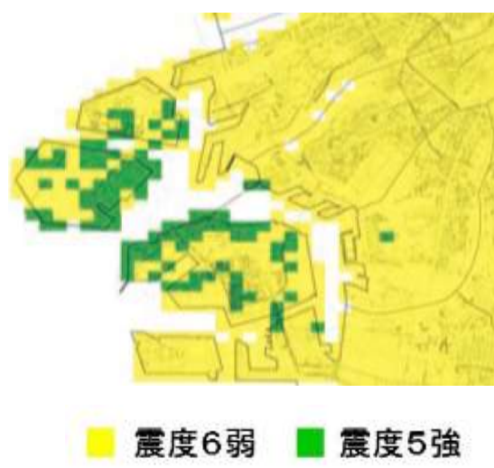
図 3-1 震度分布図
