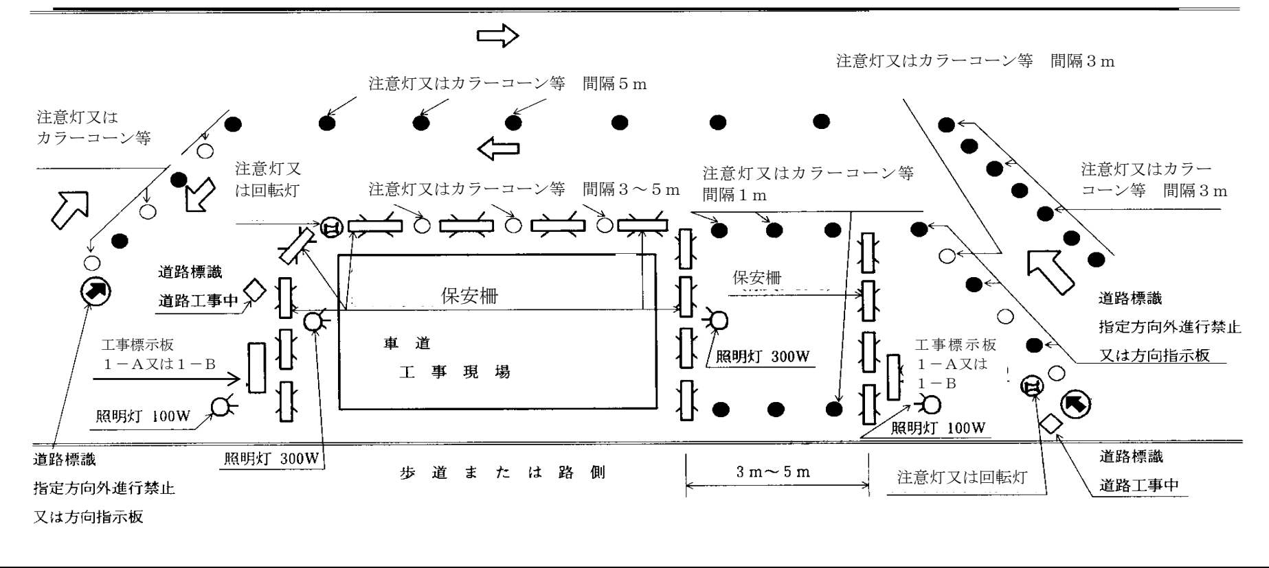
保安施設の設置例 (C) 歩道又は路側に接近する場合
