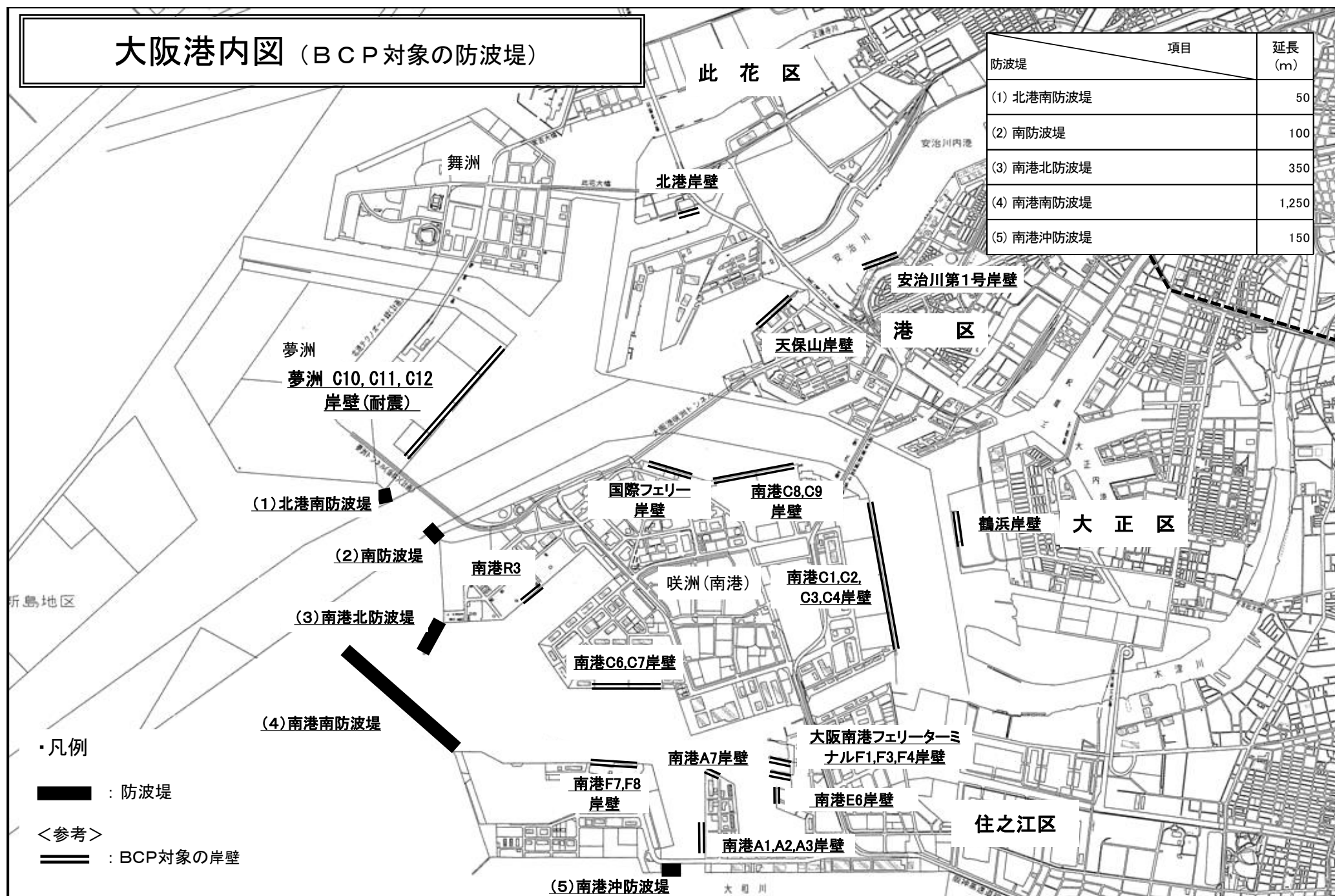
図 4-1 BCP対象の防波堤位置図
