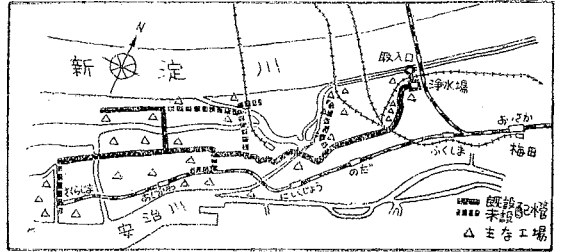
浄水場の混和池（手前）と沈澄池（向側） 下図は主要配水管図
