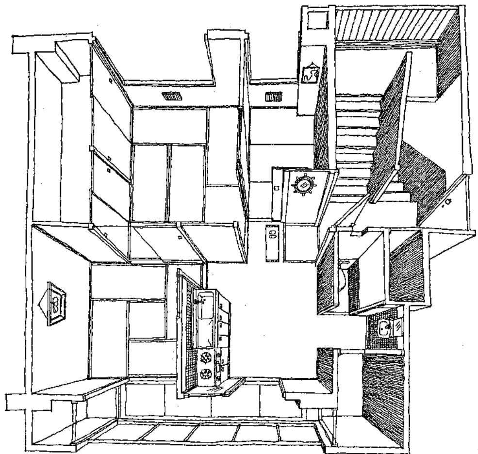
'64 3DK-A型 右上から左へ、階段・玄関・3室・6室・押入れ・4畳半・物入れ テラス・物置き(フロ場)・洗面所・トイレ・ダイニングキッチン
