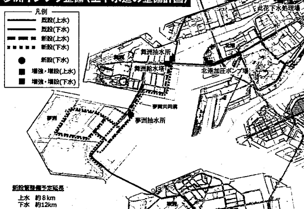
夢洲インフラ整備(上下水道の整備計画)
