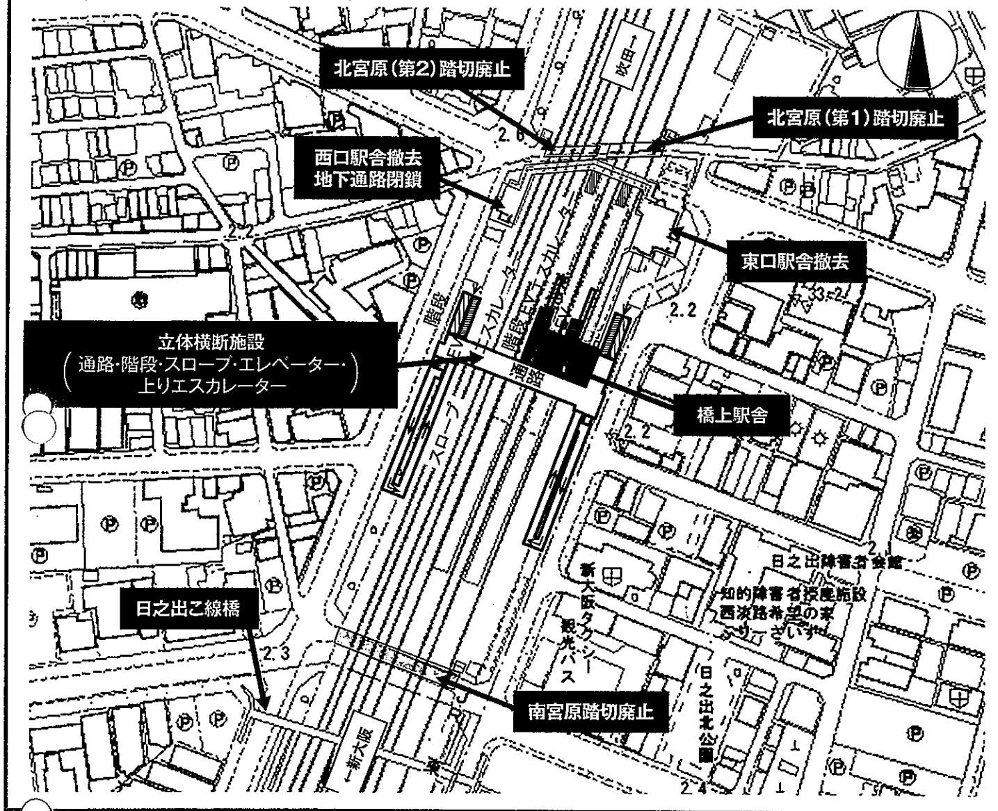
東淀川駅 立体横断施設整備工事のスケジュール (予定)
