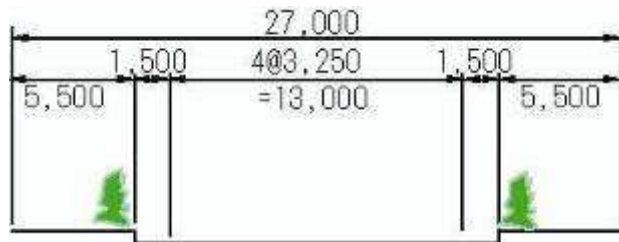
【整備断面】
