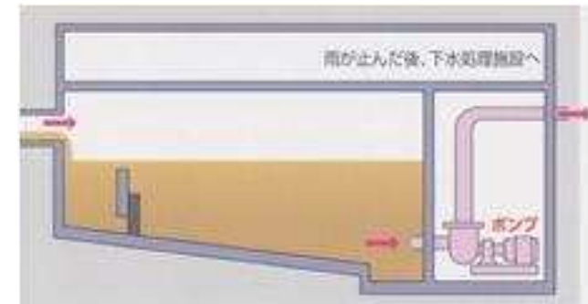
雨水滞水池
