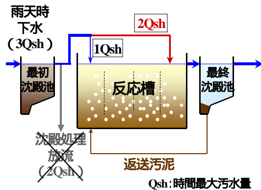
雨天時下水活性汚泥処理法
