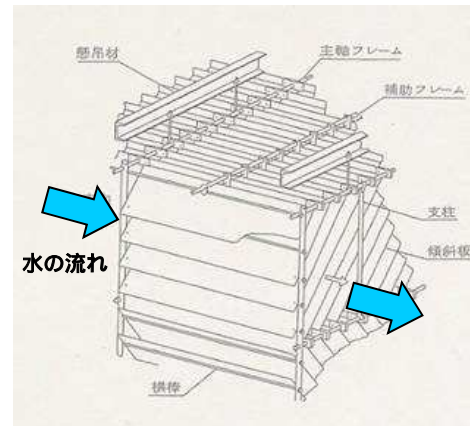
凝集傾斜板沈殿処理法
