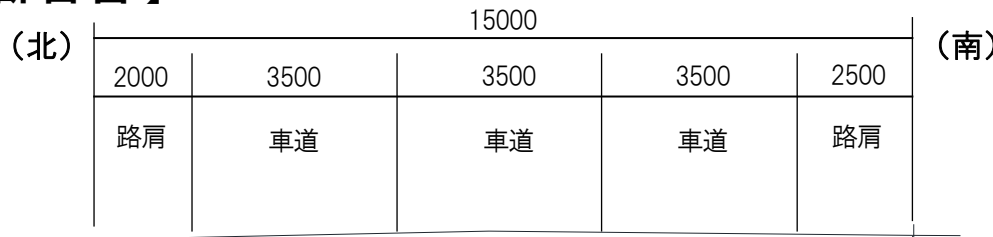
現況断面図
