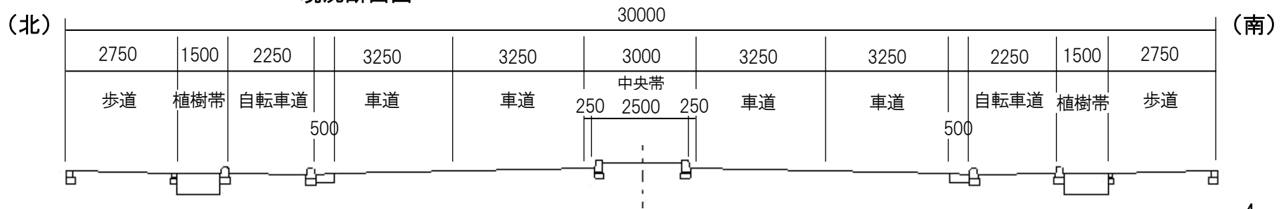
計画断面図
