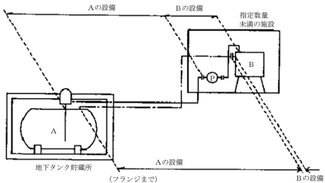
図12 配管の附属範囲の例
