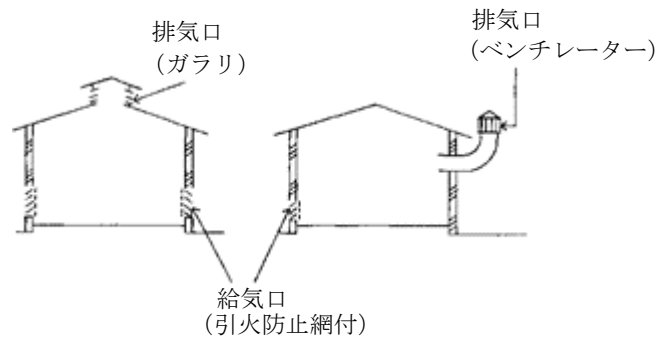
図3 換気設備の例
