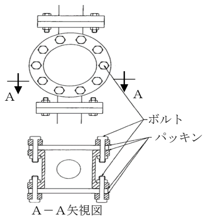
図14 蓋を設けない構造の例
