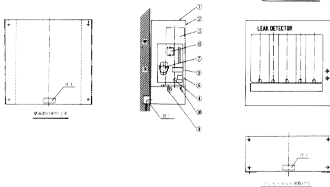
図 6-3 漏れ検知装置の例（5 タンクの場合）
