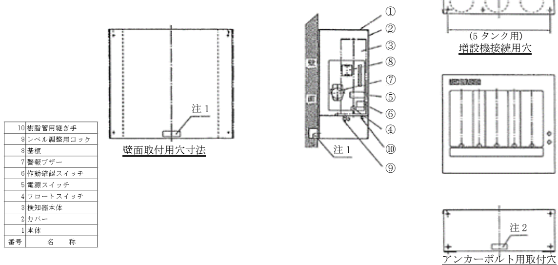
図5 タンクを複数設置した場合の漏えい検知装置の例
