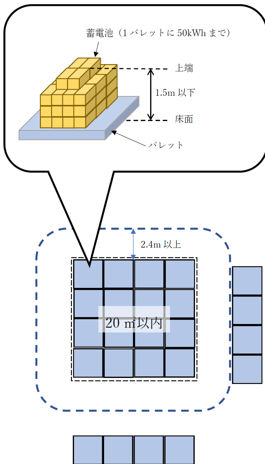
図1 規則16条の2の8第2項第5号ハによる貯蔵方法の例
