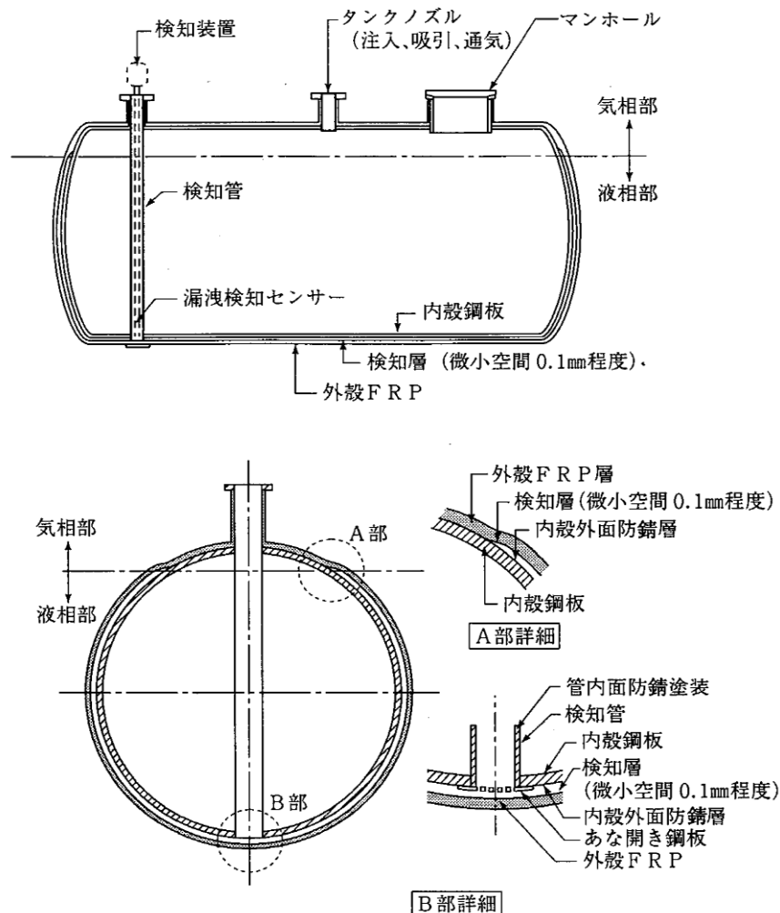
図6 鋼製強化プラスチック製二重殻タンクの構造例
