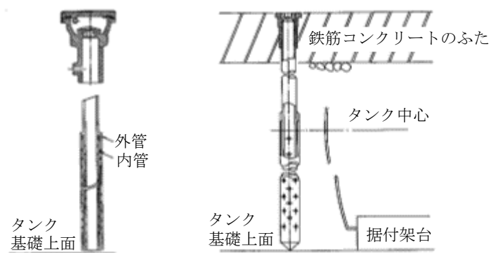
図2 漏えい検査管の構造及び設置例
