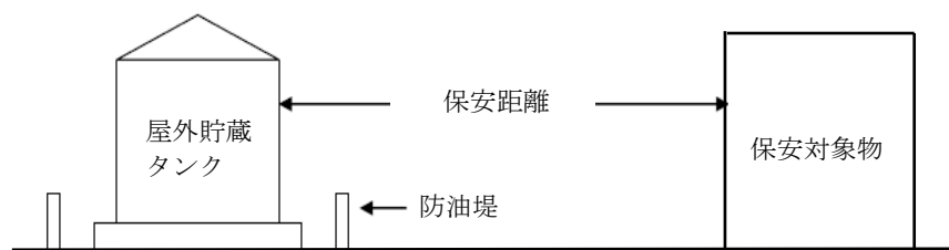
図1 保安距離の起点
