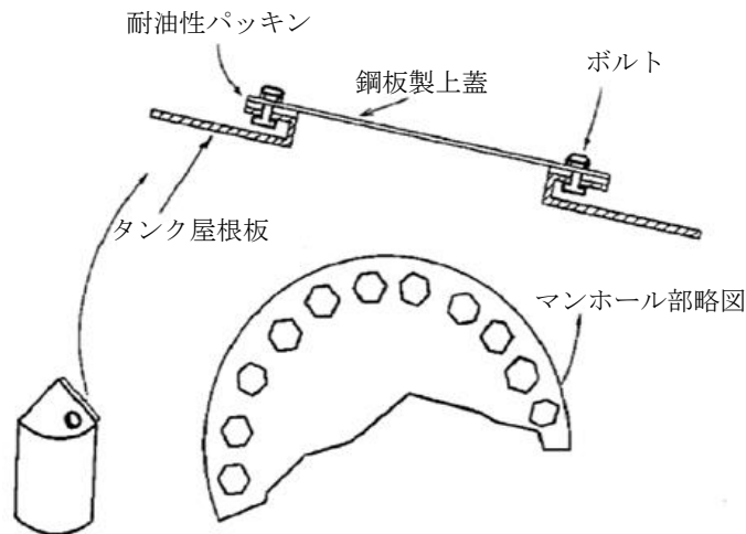
図3 気密構造の例
