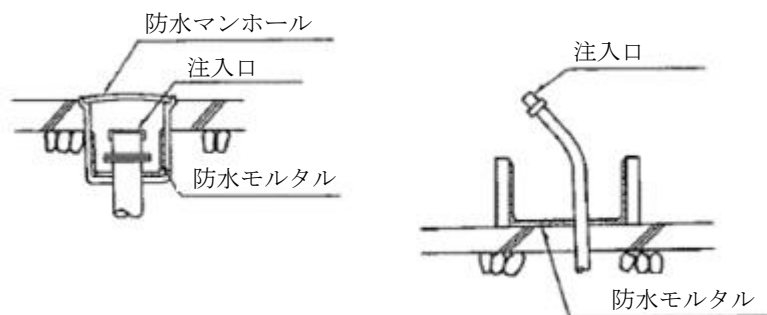
図2 措置例
