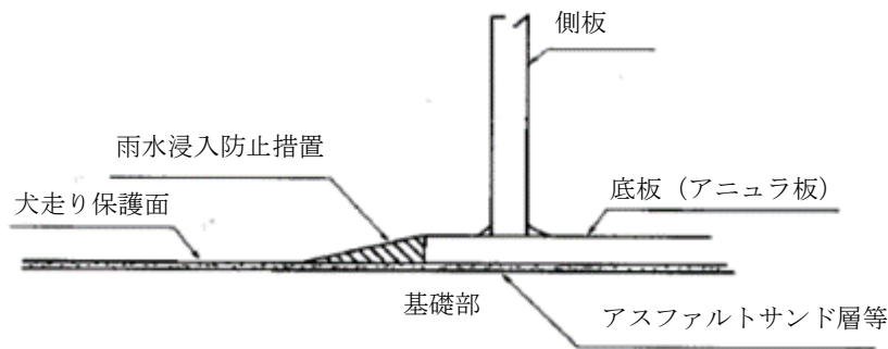
図4 被覆による措置例
