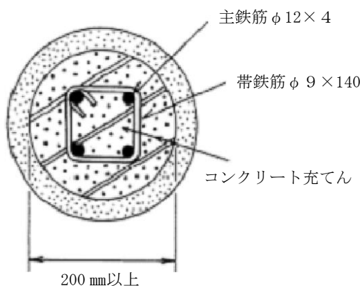
図9 鉄筋コンクリート管を用いた場合の施工例
