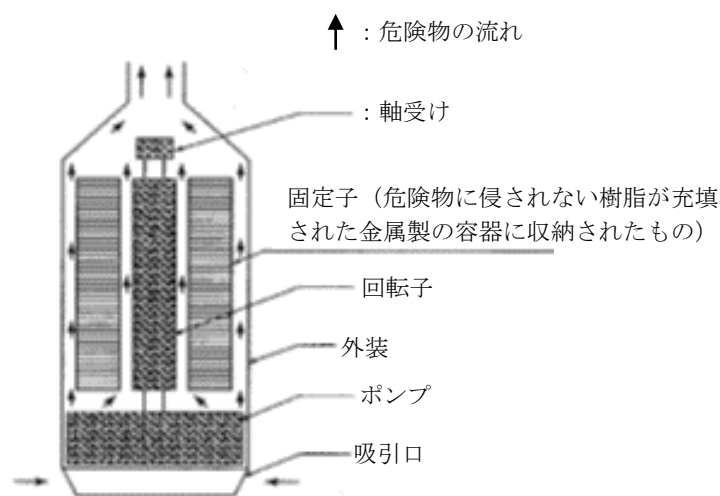
(油中ポンプ設備の模式図 (電動機の内部に危険物を通過させる場合))
