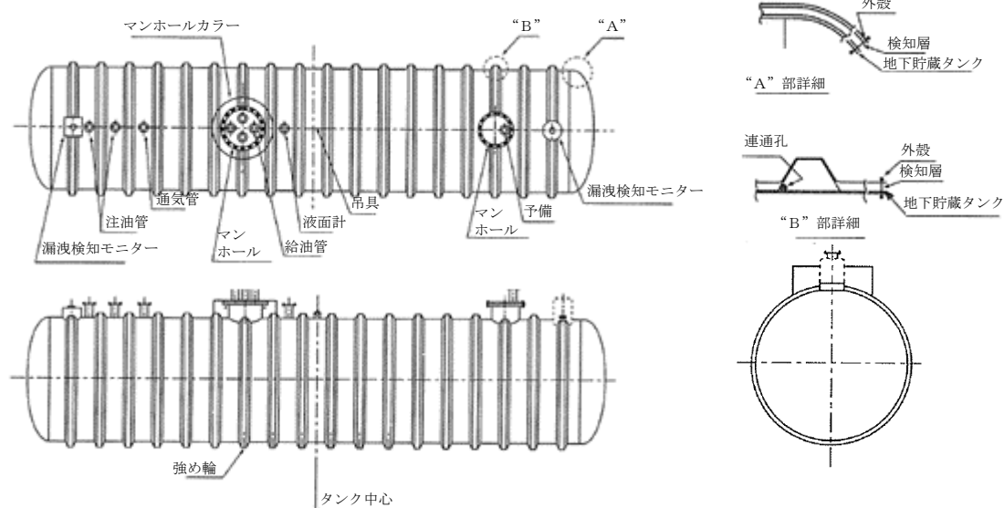
図8 強化プラスチック製二重殻タンクの構造例
