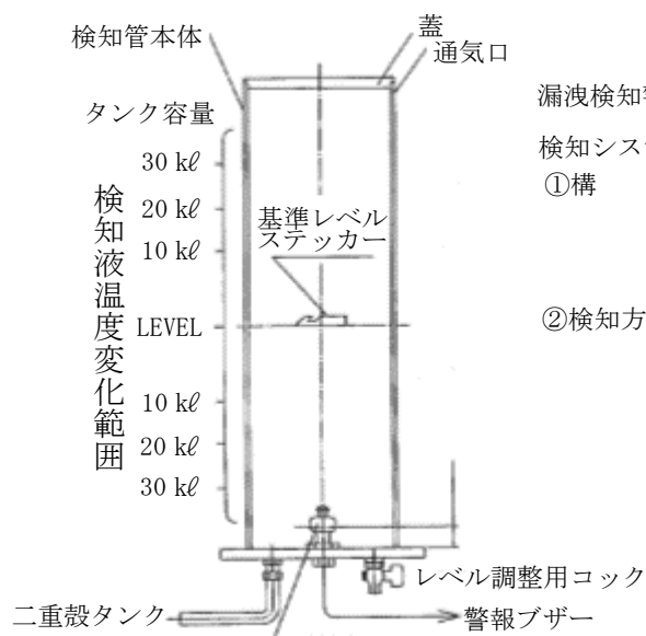
図4 漏えい検知装置の例
