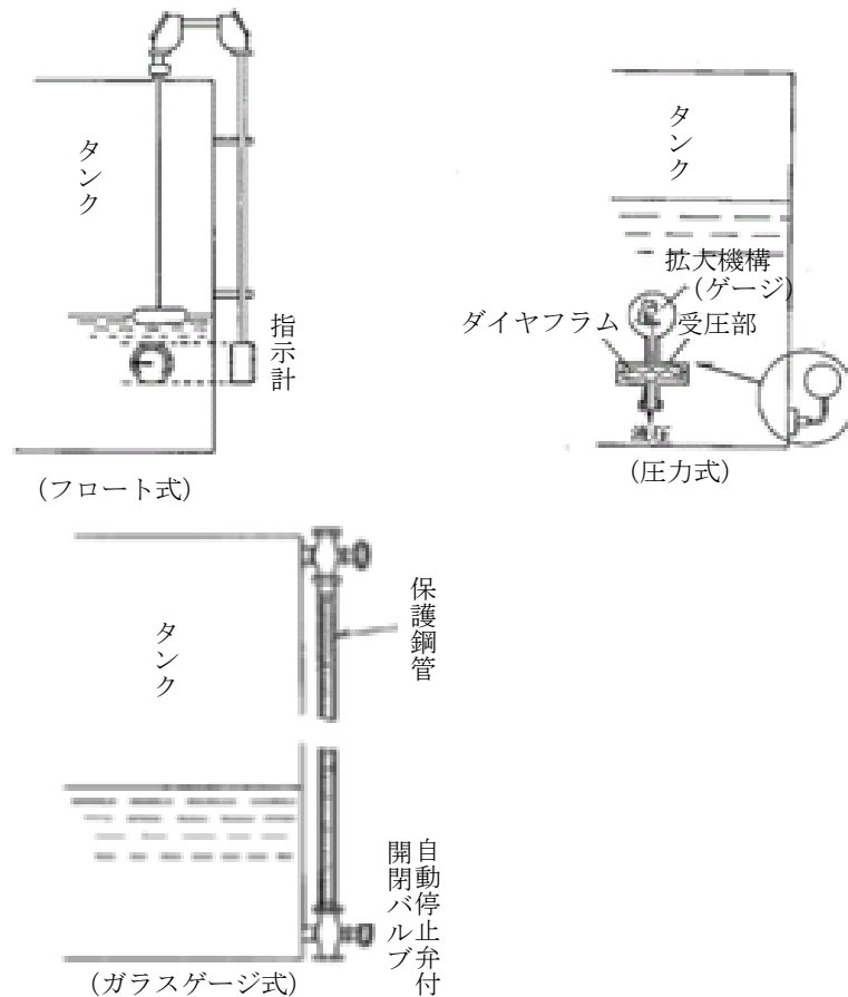
図5 自動表示装置の例
