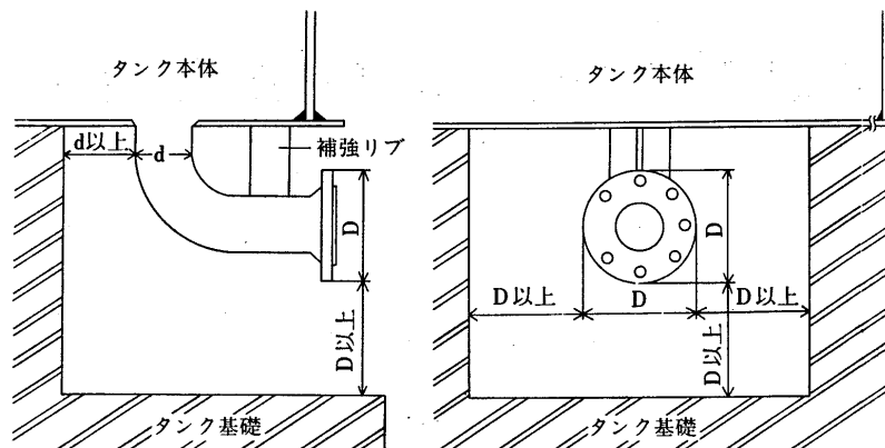
図1 水抜管の例
