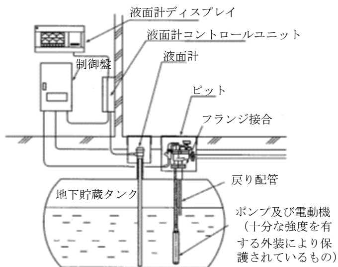
図1 油中ポンプ設備の例
