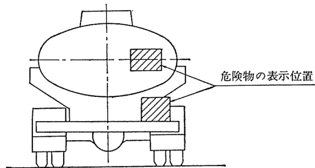
図46 表示の位置
