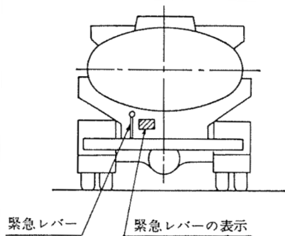
図38 緊急レバーの表示位置の例
