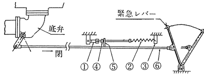
図35 自動閉鎖装置の構造
