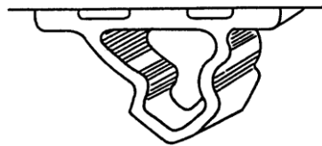
図50 計算による強度確認を行う必要のない緊締金具及びすみ金具
