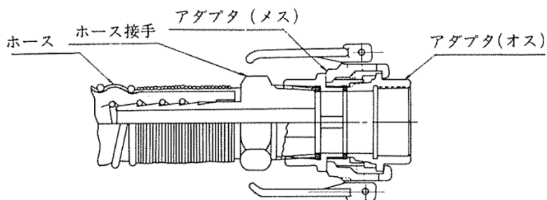
図43 突合せ固定式結合金具の構造例
