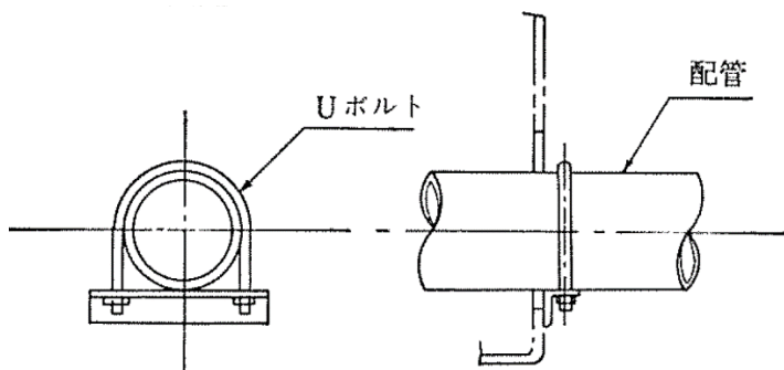
図39 配管の固定
