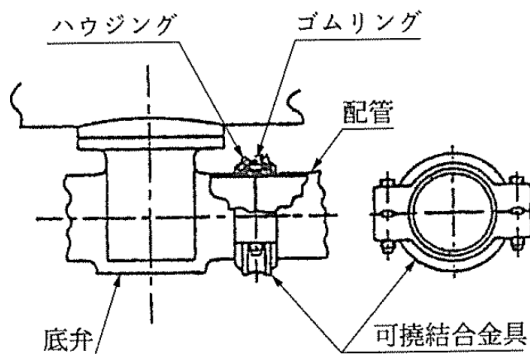
図41 緩衝用継手による方法
