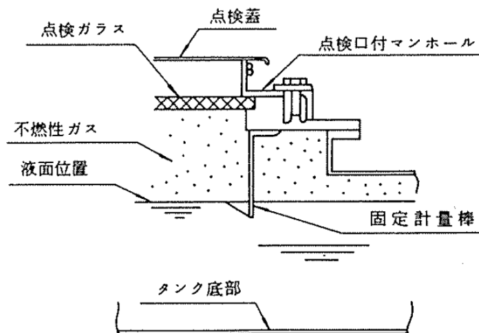
図45 静電気除去装置の構造の例
