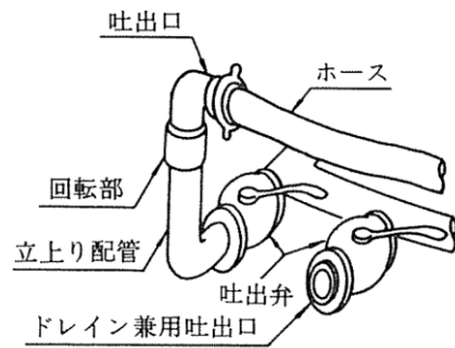
図44 配管先端部の構造例
