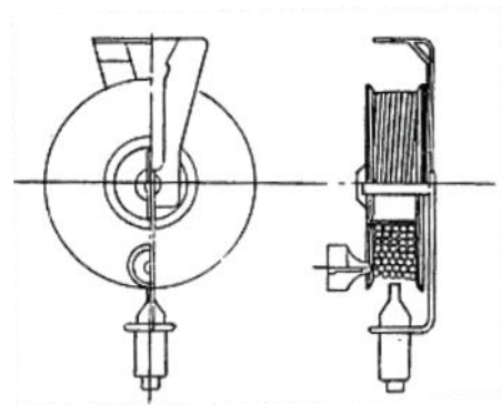
図42 巻取り装置の例
