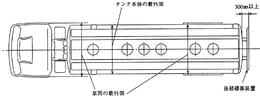
図49 最大容量が20キロリットルを超える移動タンク貯蔵所のタンクの位置
