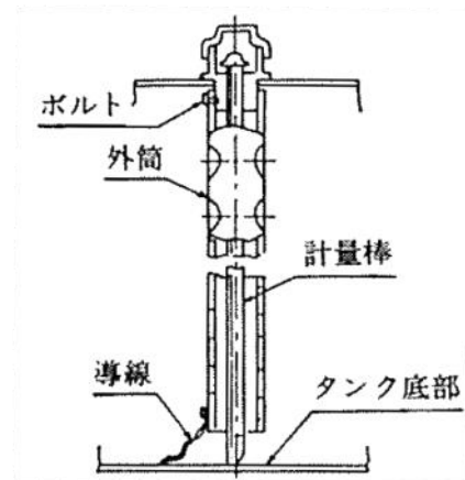
例4 外筒を上下の受け金で 取り付ける例
