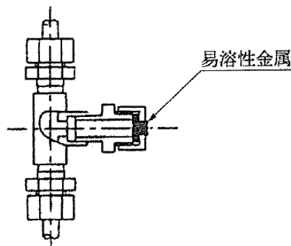
図37 熱感知部分の構造
