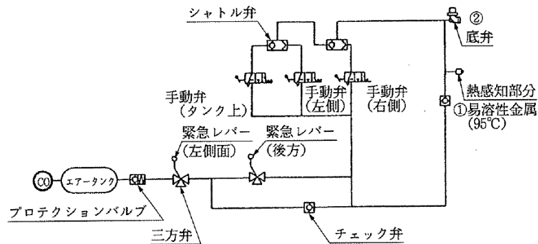
図36 底弁の自動閉鎖の系統図
