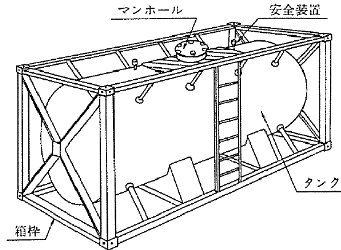
図51 箱枠の例
