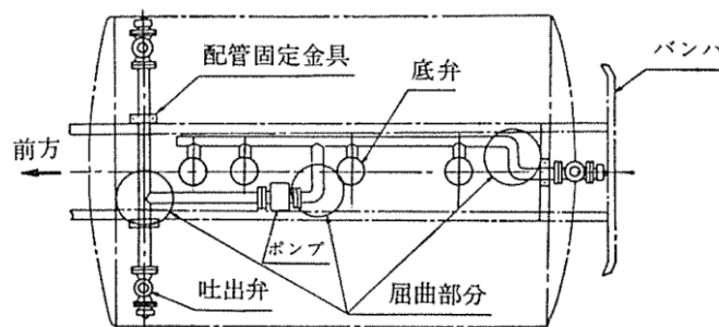
図40 配管による方法
