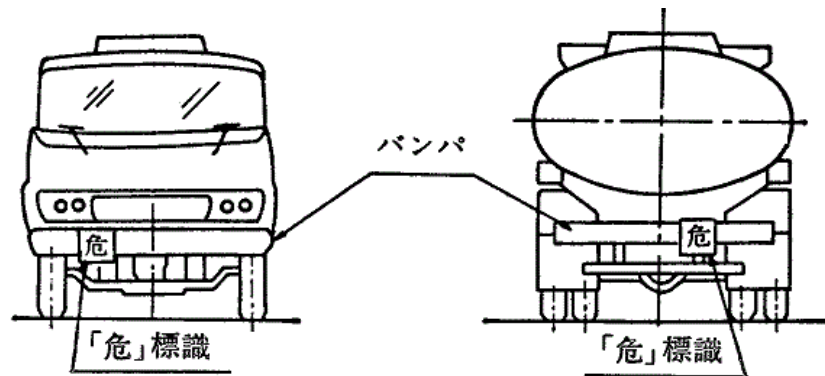
図47 標識の取付位置
