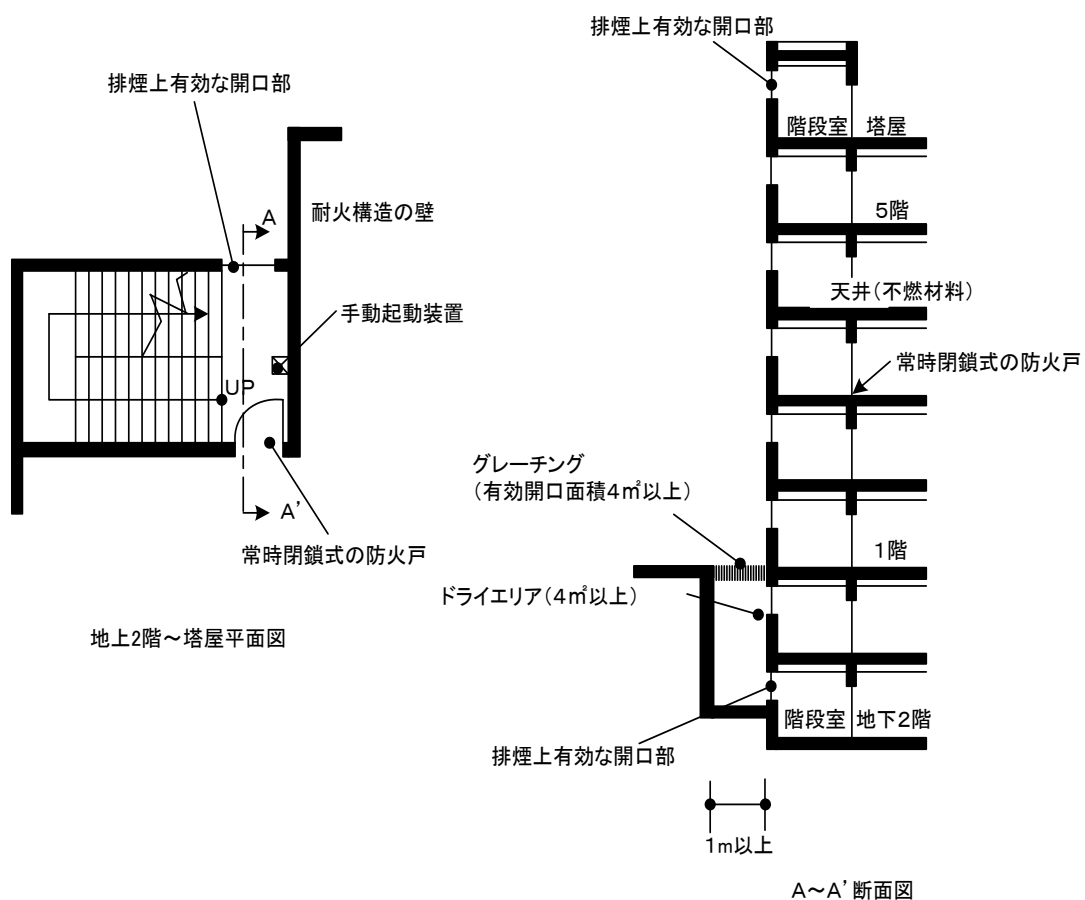
A~A' 断面図
