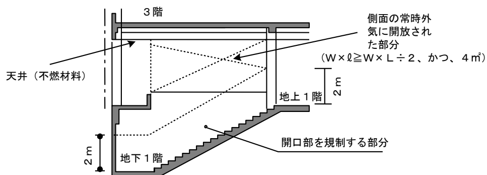
A~A' 断面图
