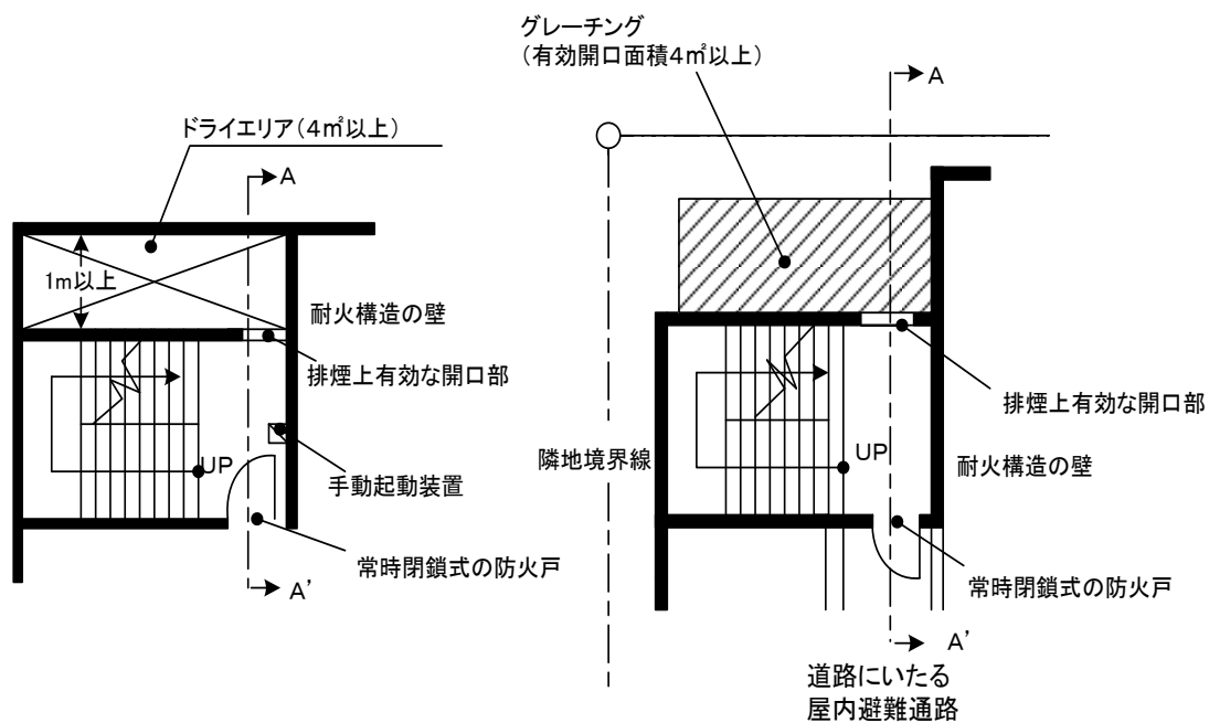
地下1階、地下2階平面図
