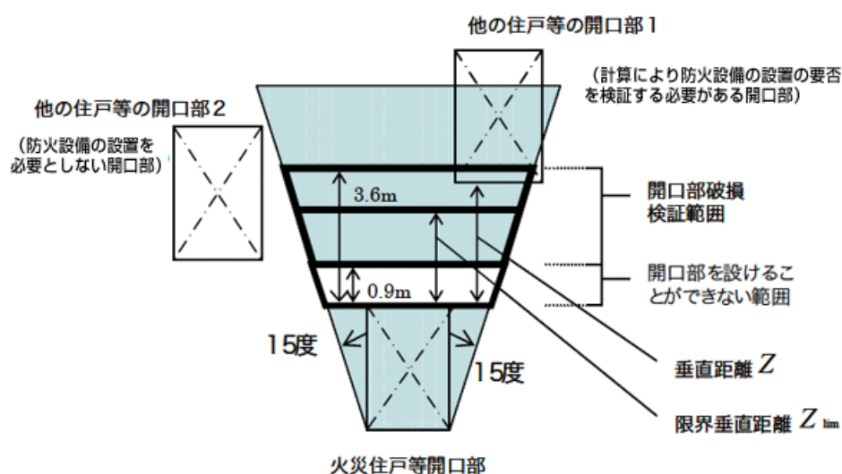
火災住戸等の開口部から噴出する火炎の影響を考慮すべき範囲
