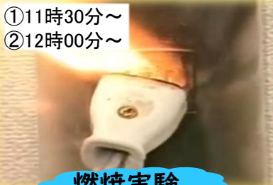
燃焼実験
