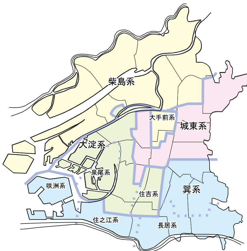
図4 大阪市の配水系統図
