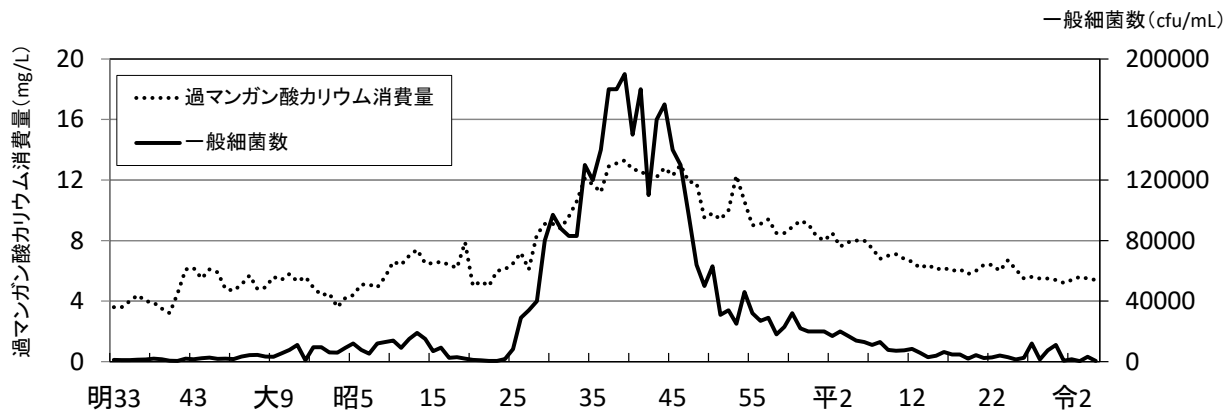
図2 柴島浄水場原水水質の変遷
