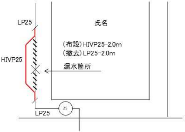
修 繕 図
