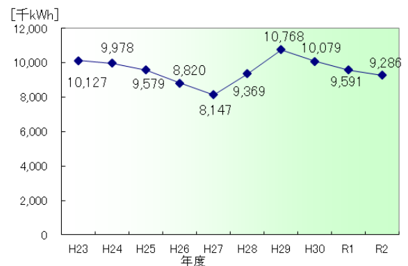
【オゾン注入制御の改良による過去 10 年間の電力削減量】
