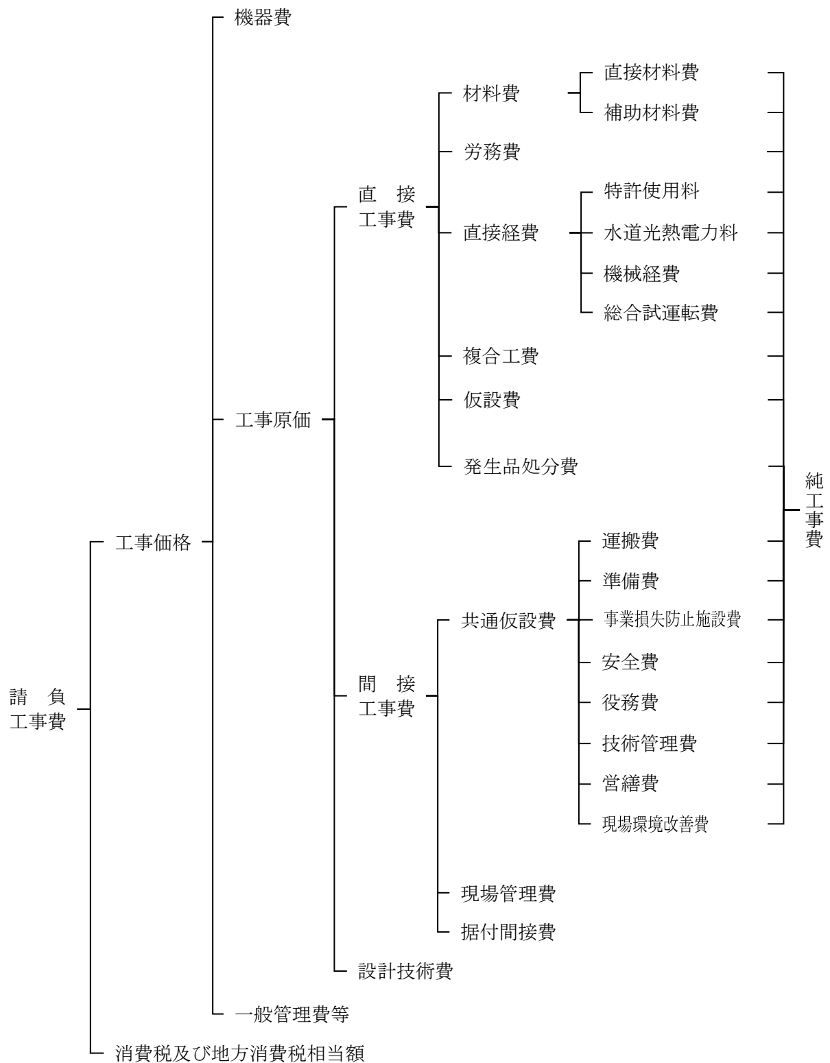
図－１ 請負工事費の構成
