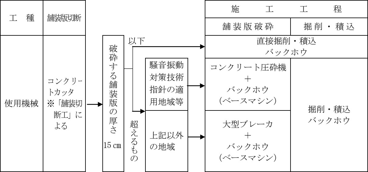
図2-1 機種の選定
