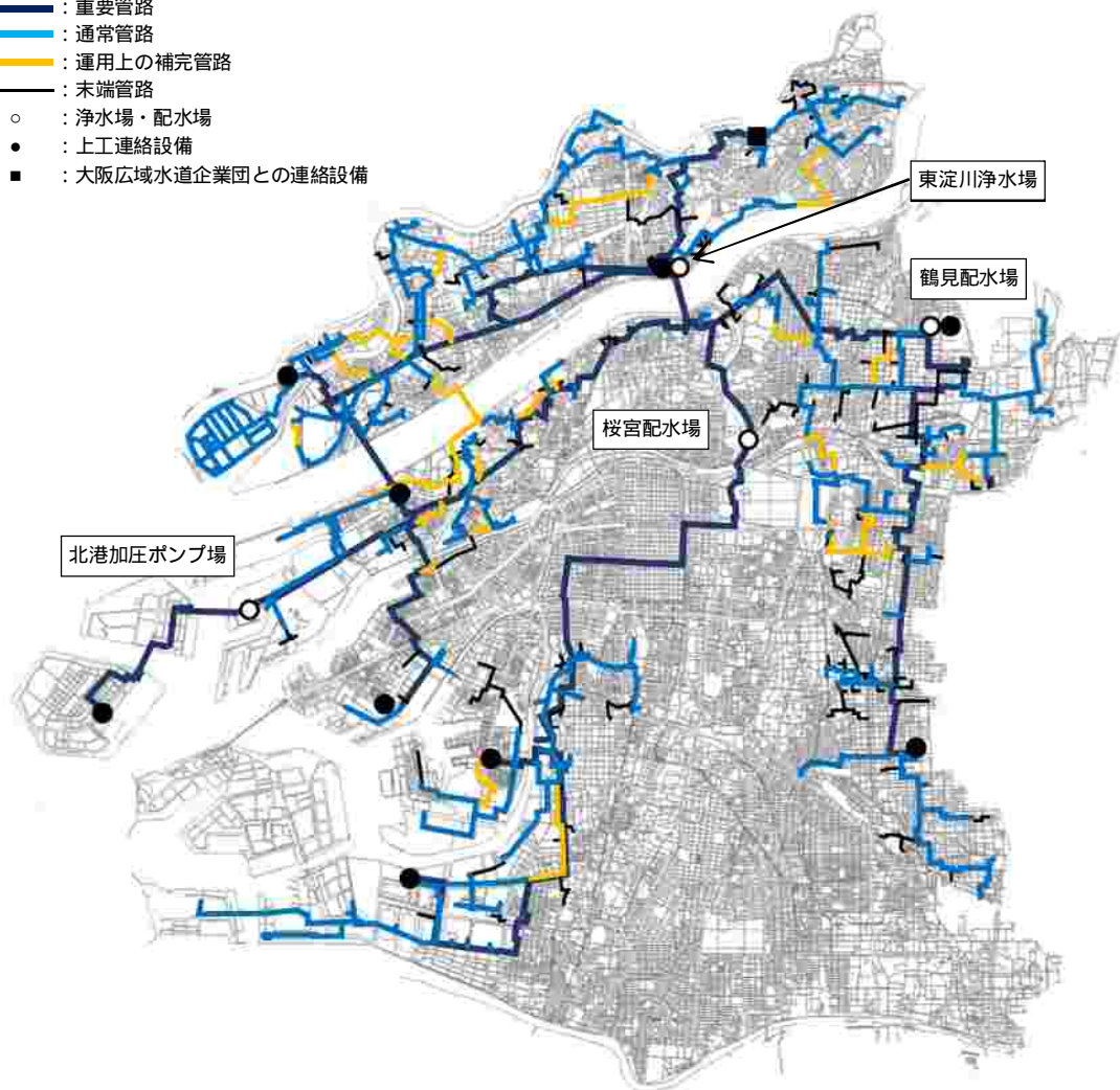
図 4 - 2 工業用水道管路の機能分類：位置図（2020 年 10 月 1 日時点）
