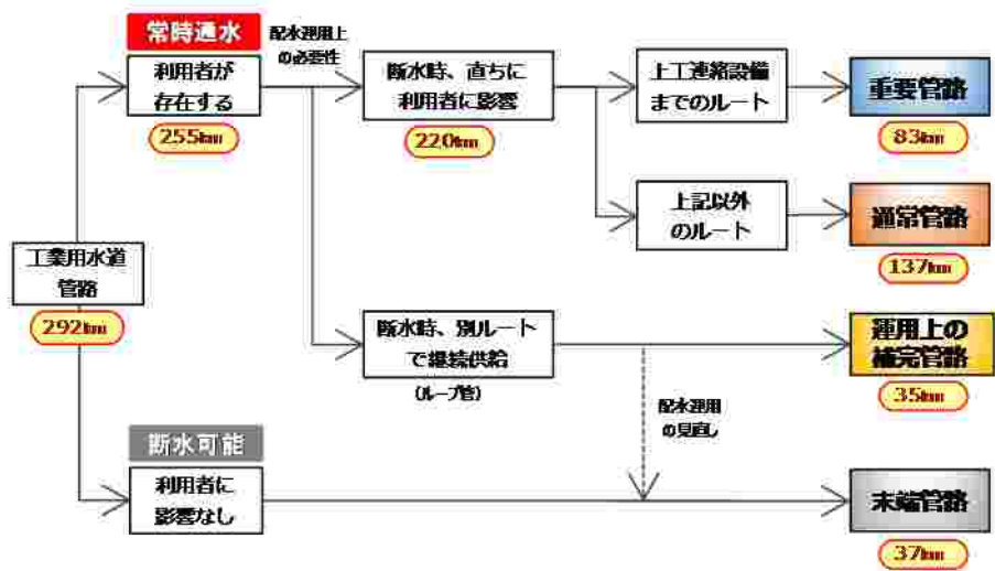
図 4 - 1 工業用水道管路の機能分類：概念図（2020 年 10 月 1 日時点）
