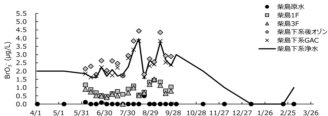
図-1 柴島下系処理過程の臭素酸濃度
