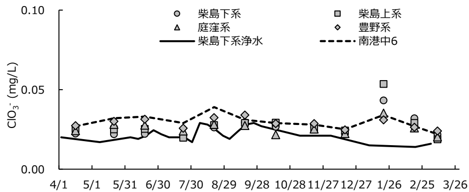
図-7 市内給水栓における塩素酸濃度
