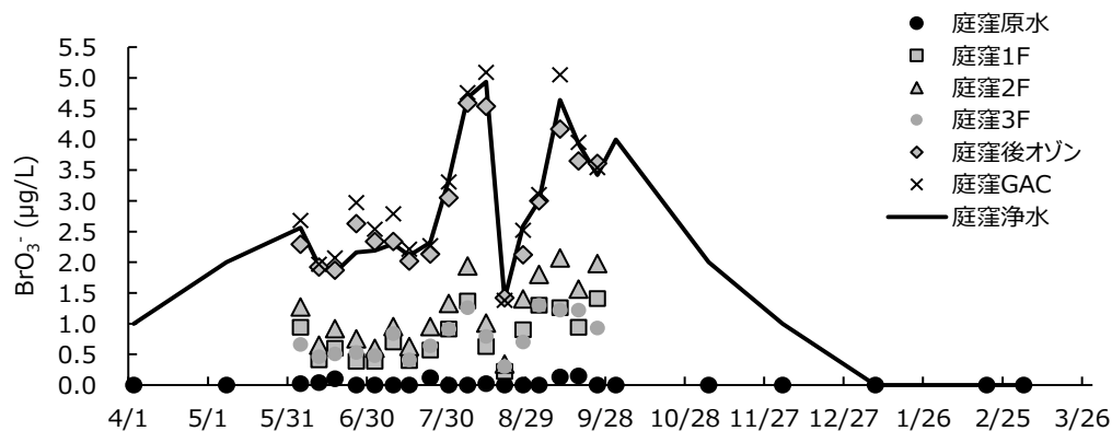
図-3 庭窪系処理過程の臭素酸濃度
