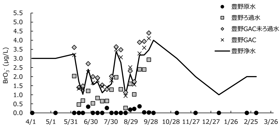
図-4 豊野系処理過程の臭素酸濃度
