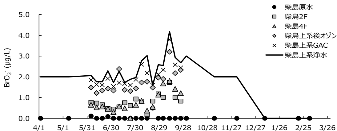
図-2 柴島上系処理過程の臭素酸濃度
