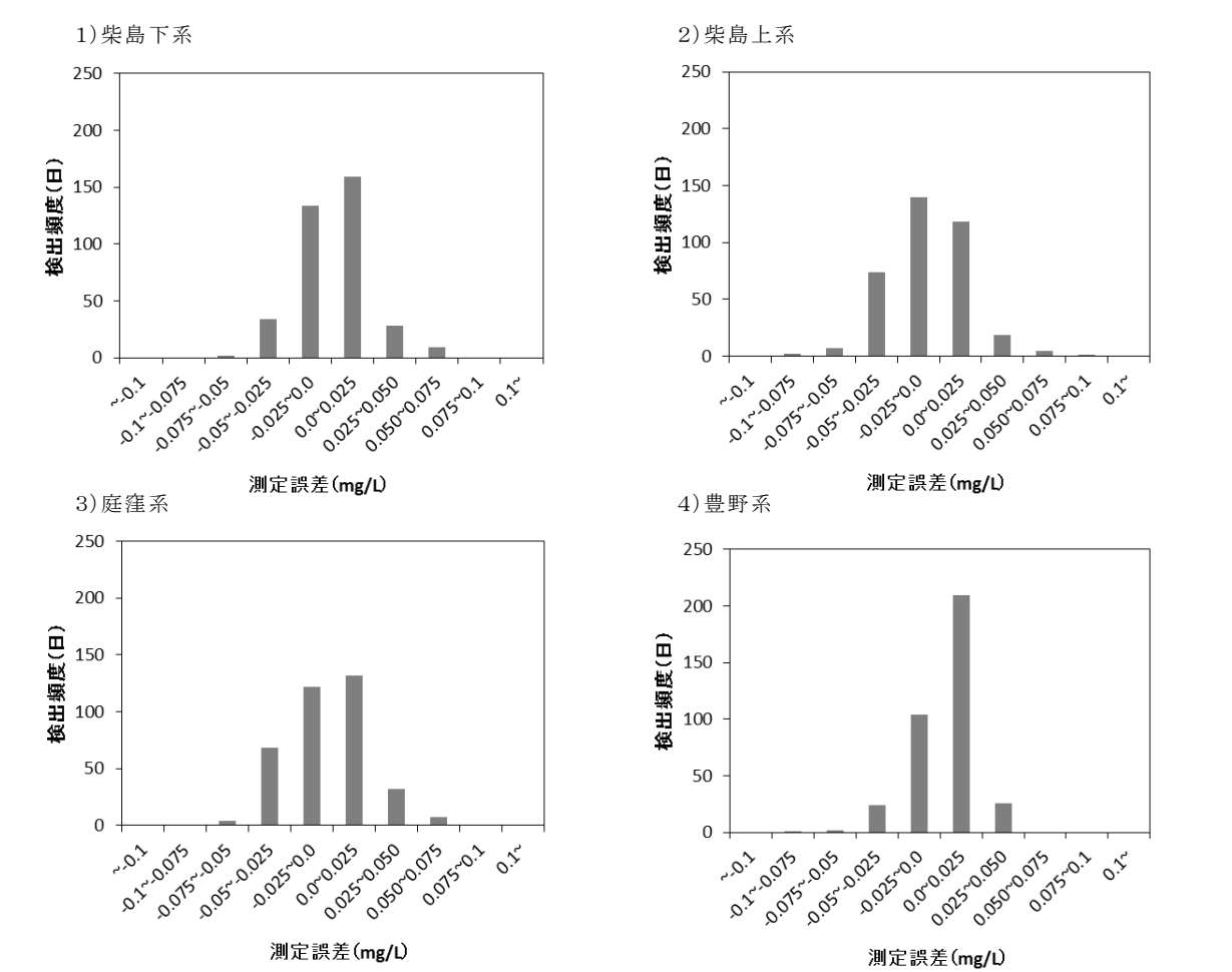
図-2 各配水系統における測定誤差の分布
