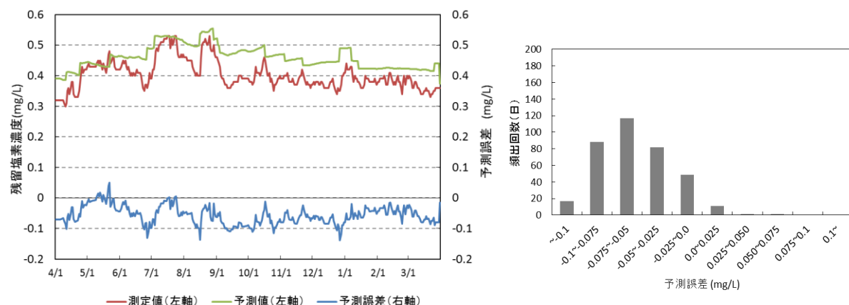
図-3 各配水系統における水質 TM の予測値と実測値との濃度差の推移と分布
