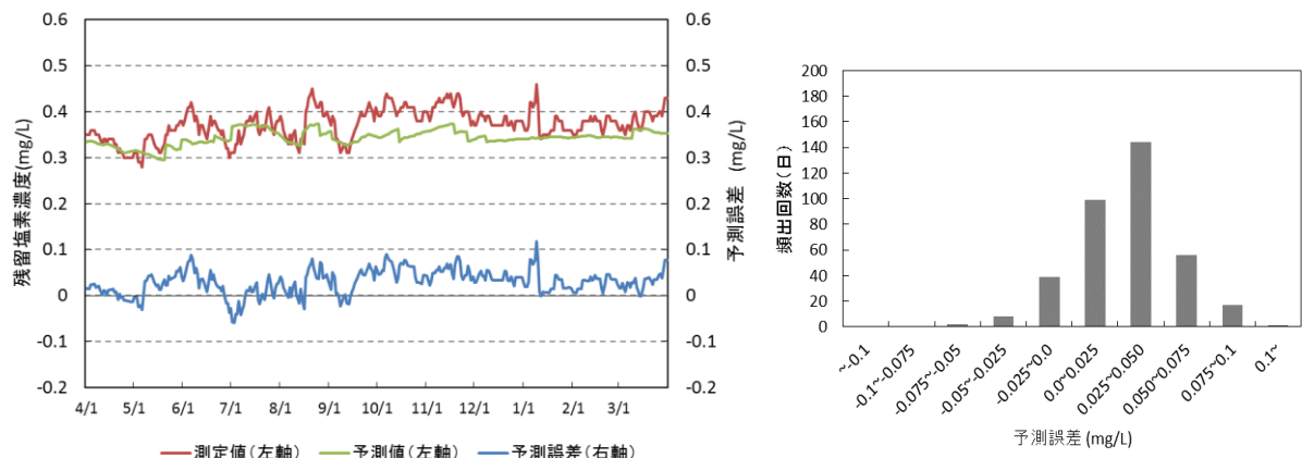
図-3 各配水系統における水質 TM の予測値と実測値との濃度差の推移と分布（つづき）
