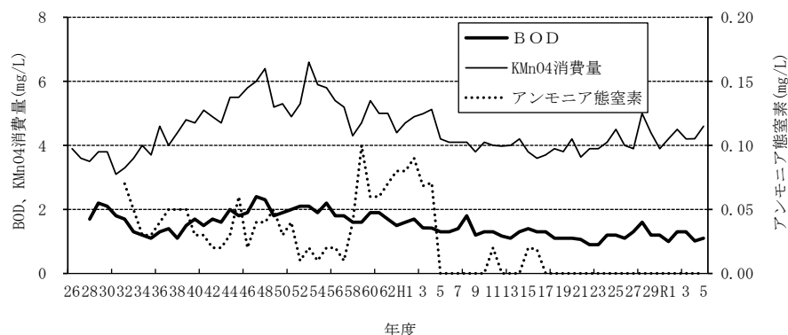
図1-3-1 琵琶湖（三井寺沖）水質の経年変化
