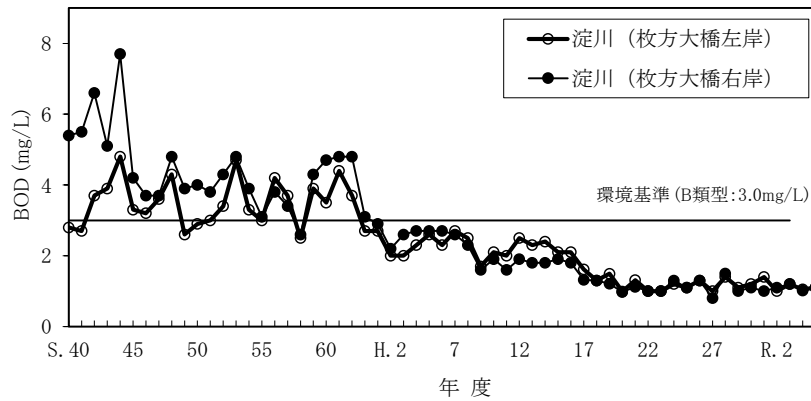
図2-2-2 枚方地点におけるBODの経年変化
