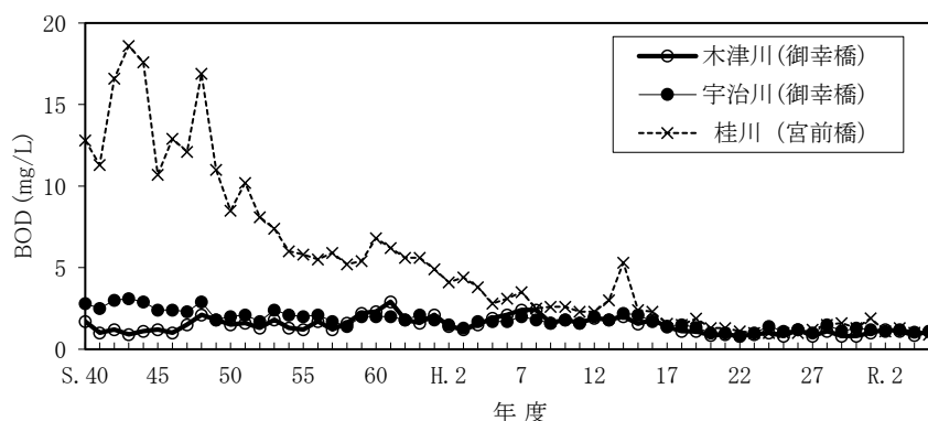
図2-2-1 三川におけるBODの経年変化
