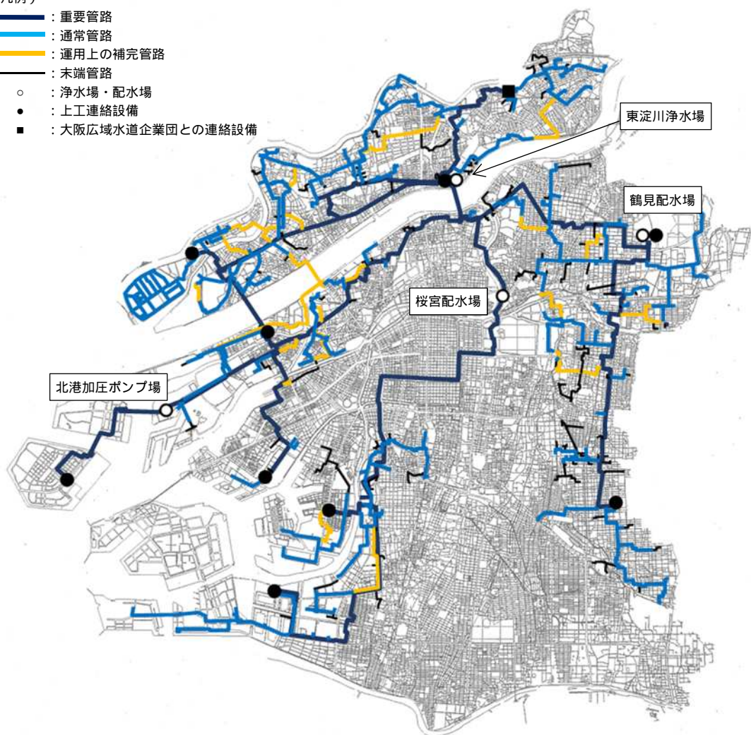
図 4 - 2 工業用水道管路の機能分類：位置図（2022 年 3 月 1 日時点）
