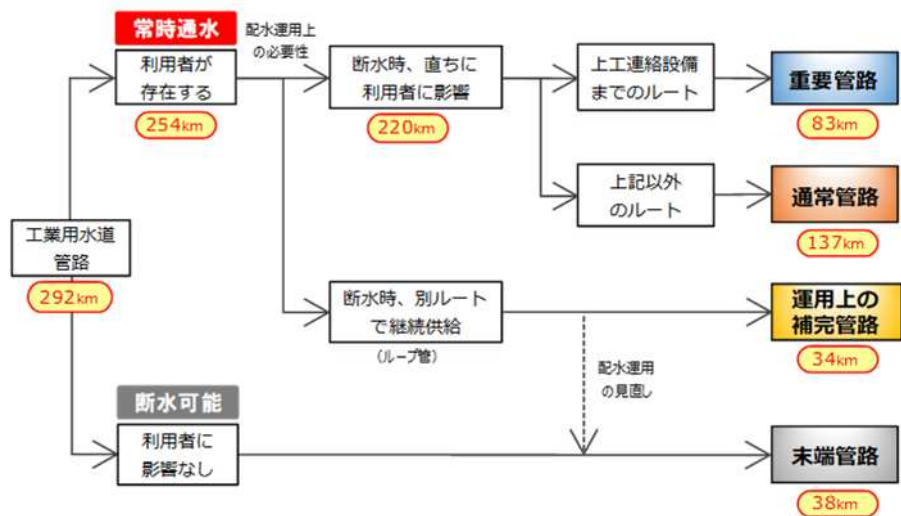
図 4 - 1 工業用水道管路の機能分類：概念図（2022 年 3 月 1 日時点）
