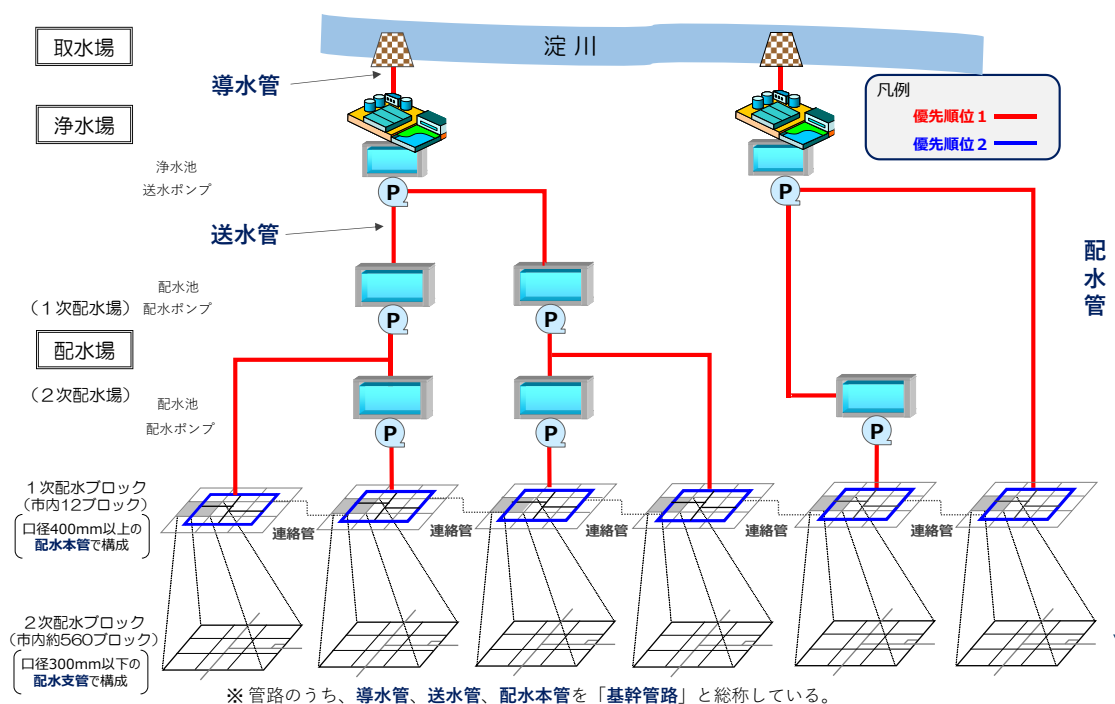
図表6-1 上町断層帯地震に対する管路整備の優先順位
