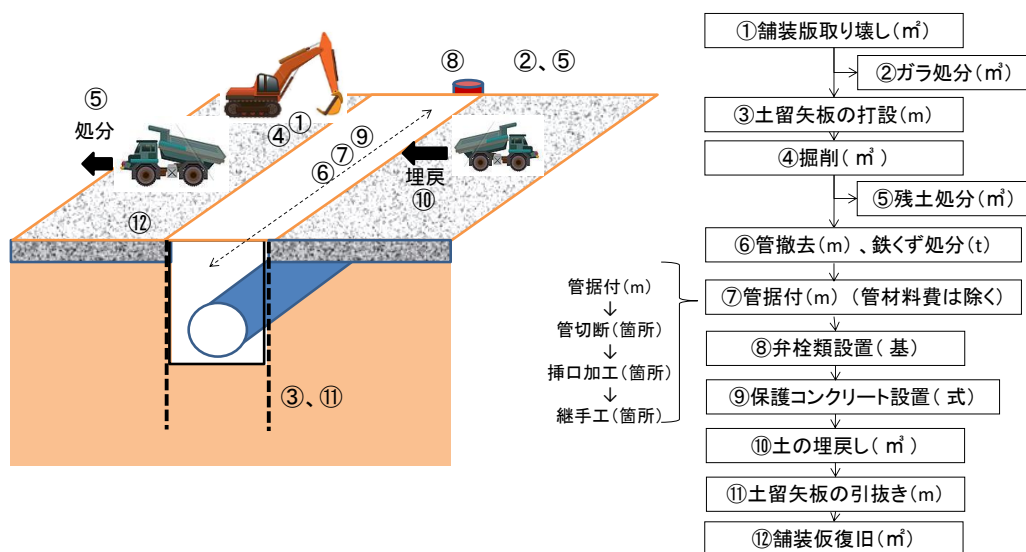
図3 基礎的工種を構成する主な工種
