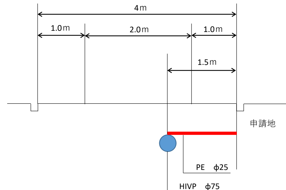
断面図
