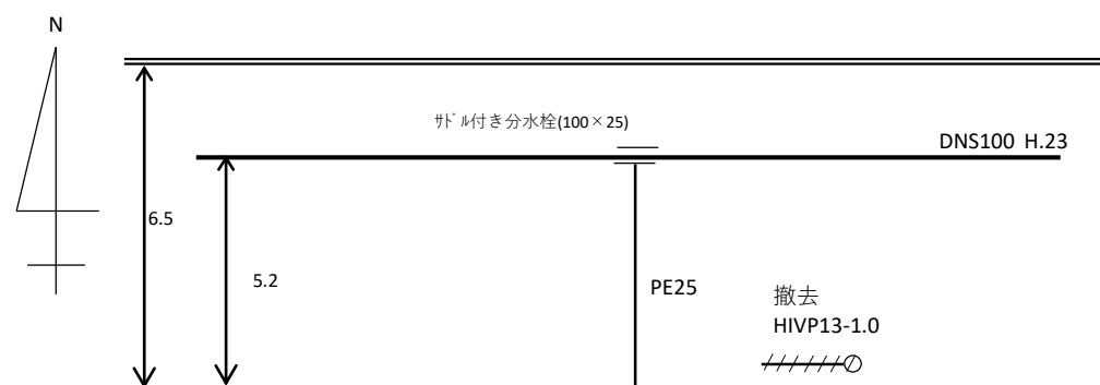
給水装置工事図面
