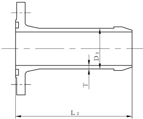
S 5 0 形短管 2 号
