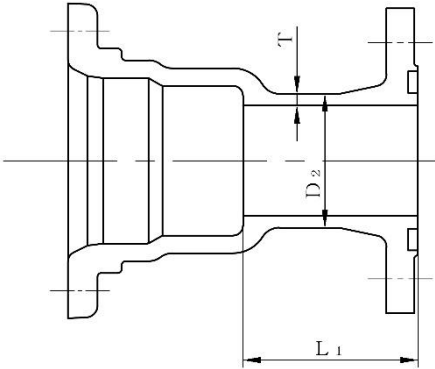
S 5 0 形短管 1 号
